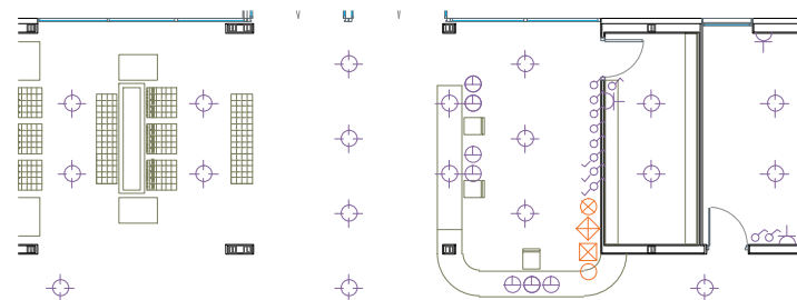
Conserjería y área de espera planta Baja _e:1/100
