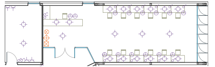
Sala informática planta Tercera _e:1/100
