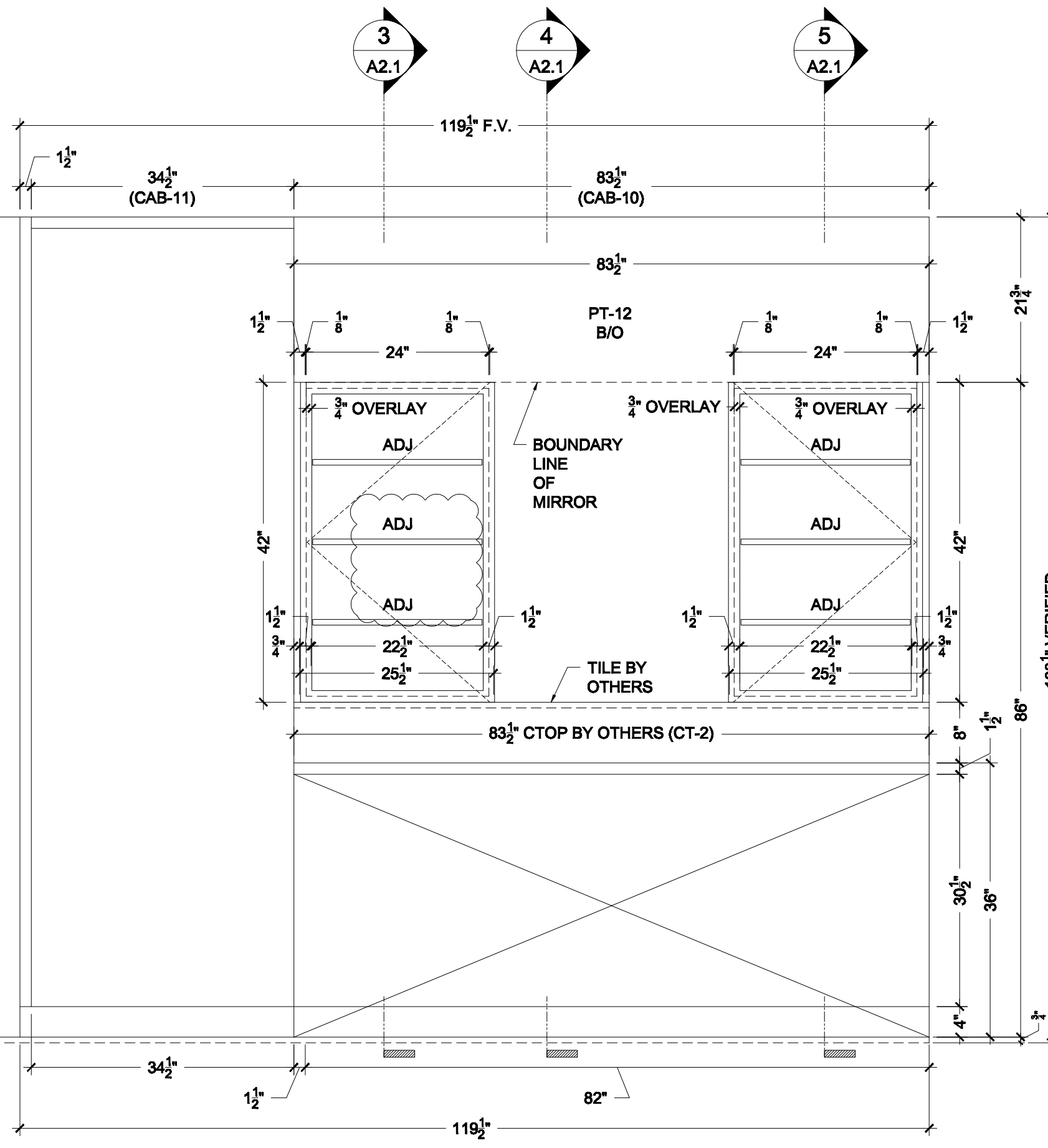
4 MIRROR LAYOUT SCALE: 3/4" = 1'-0"
