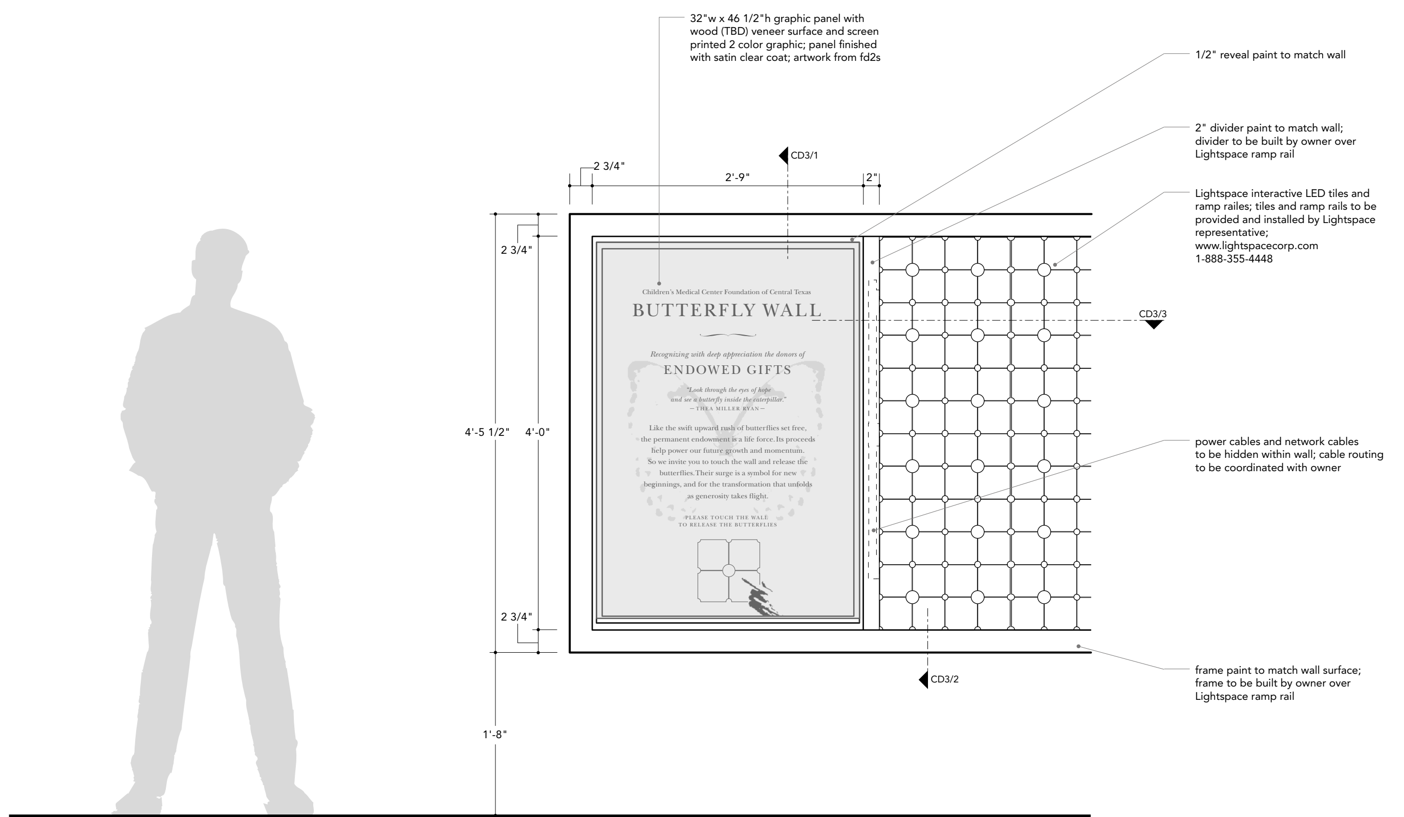
1 Elevation scale: 1"=1'-0"
