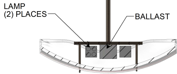
SECTION A-A SCALE 1 : 5
