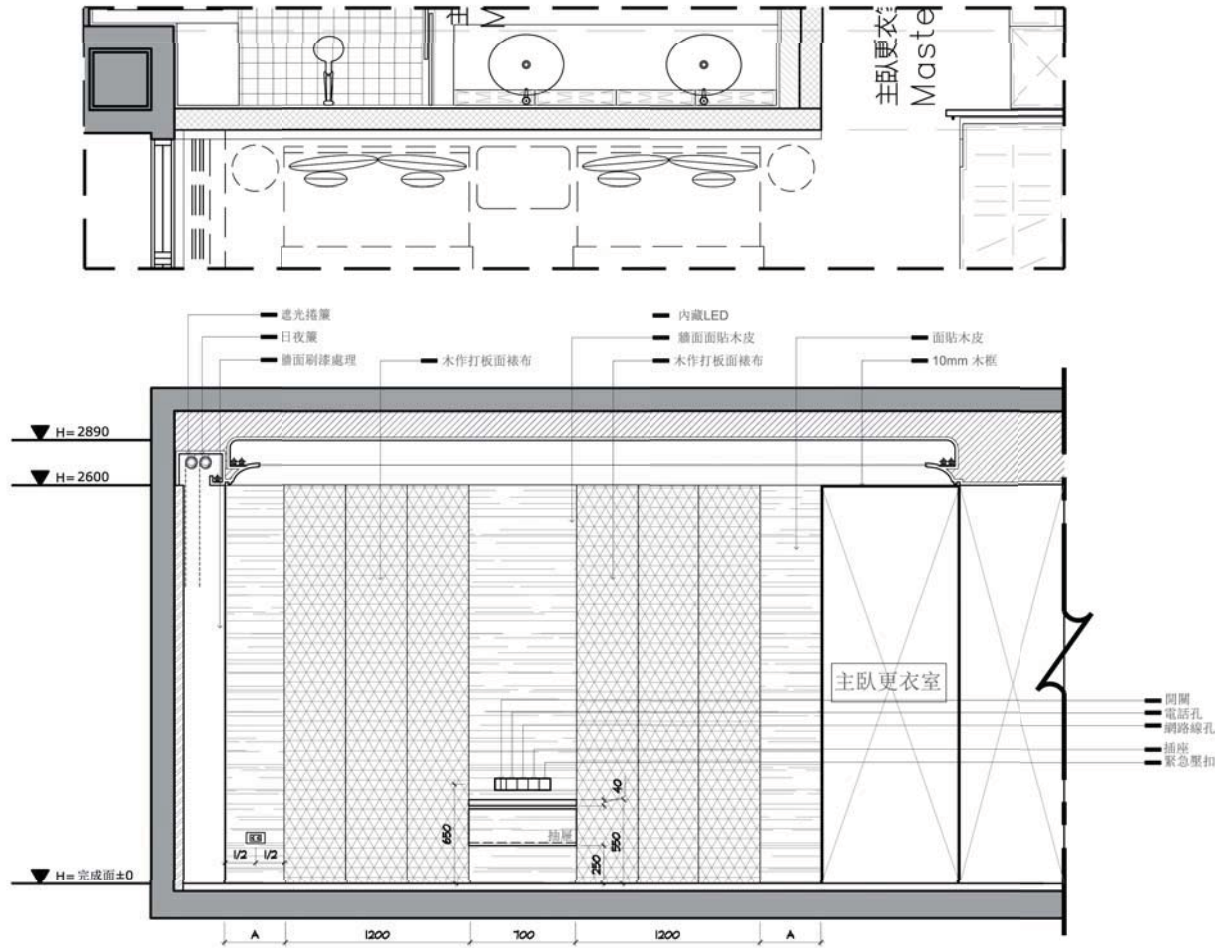
E8-B 主臥立面圖 SCALE: 1/30
