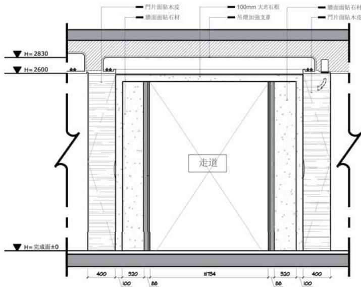
E3-B 餐廳立面圖 SCALE: 1/30
