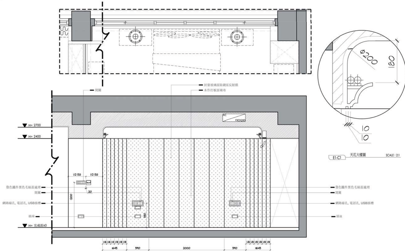
E1-C 主臥立面圖 SCALE: 1/30
