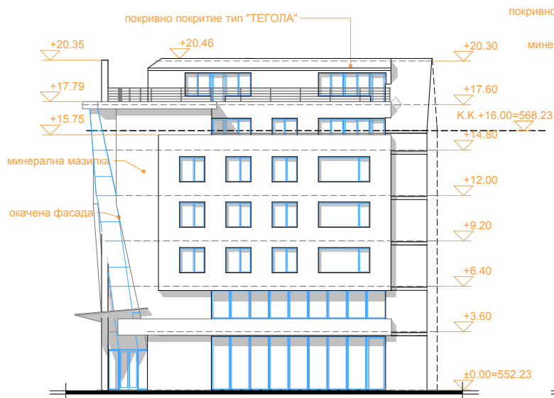
ФАСАДА СЕВЕР
