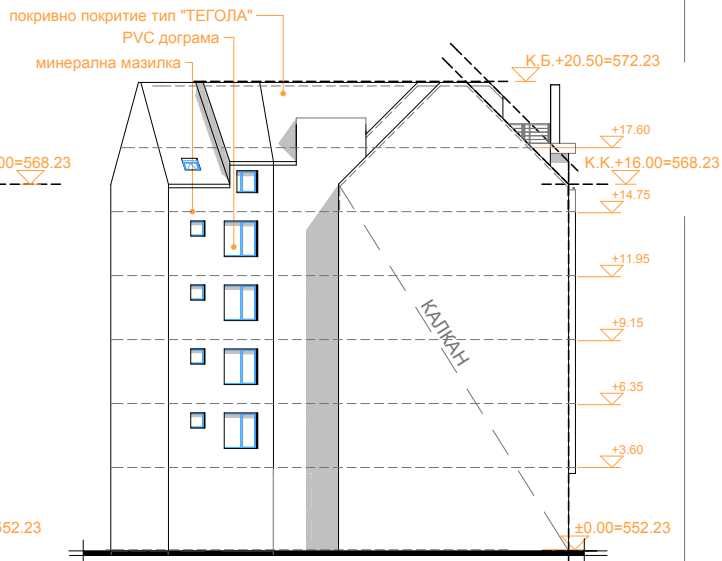
ФАСАДА ЮГ
