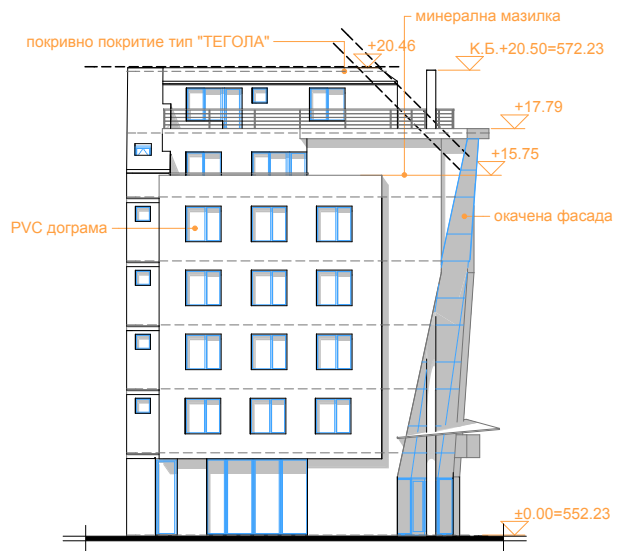
ФАСАДА ИЗТОК
