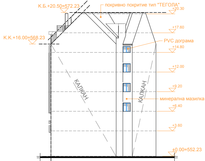
ФАСАДА ЗАПАД
