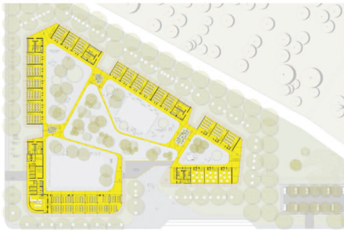
Planta nivel 0.00
