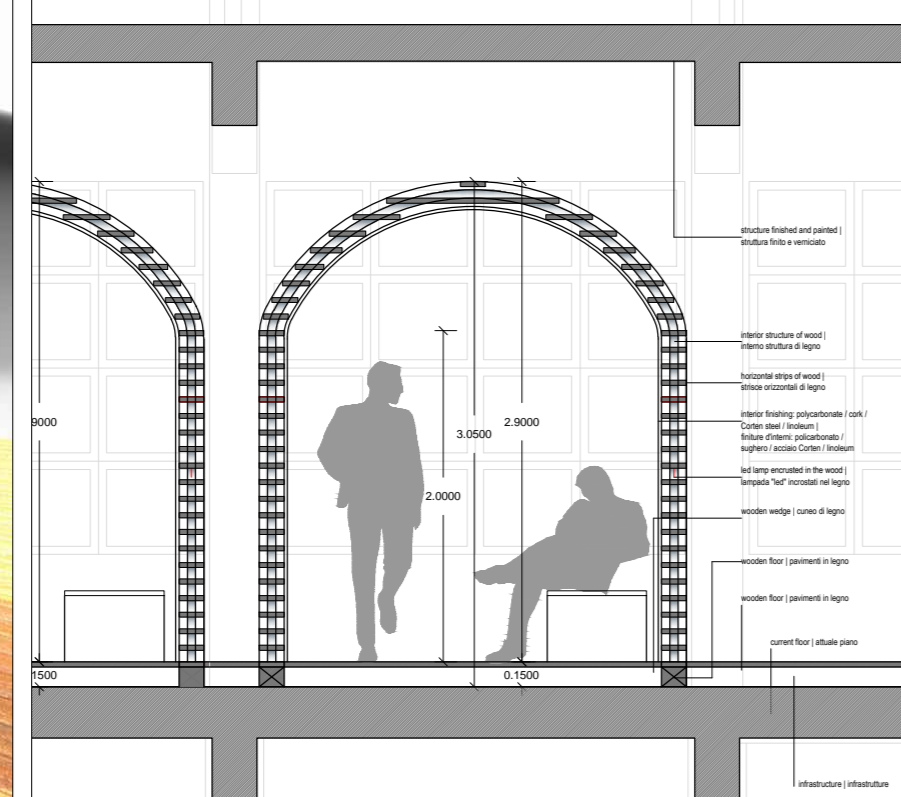
CROSS / SEZIONE
