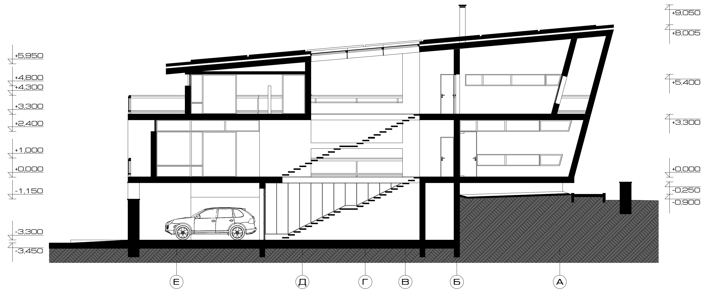
Разрез A-A
