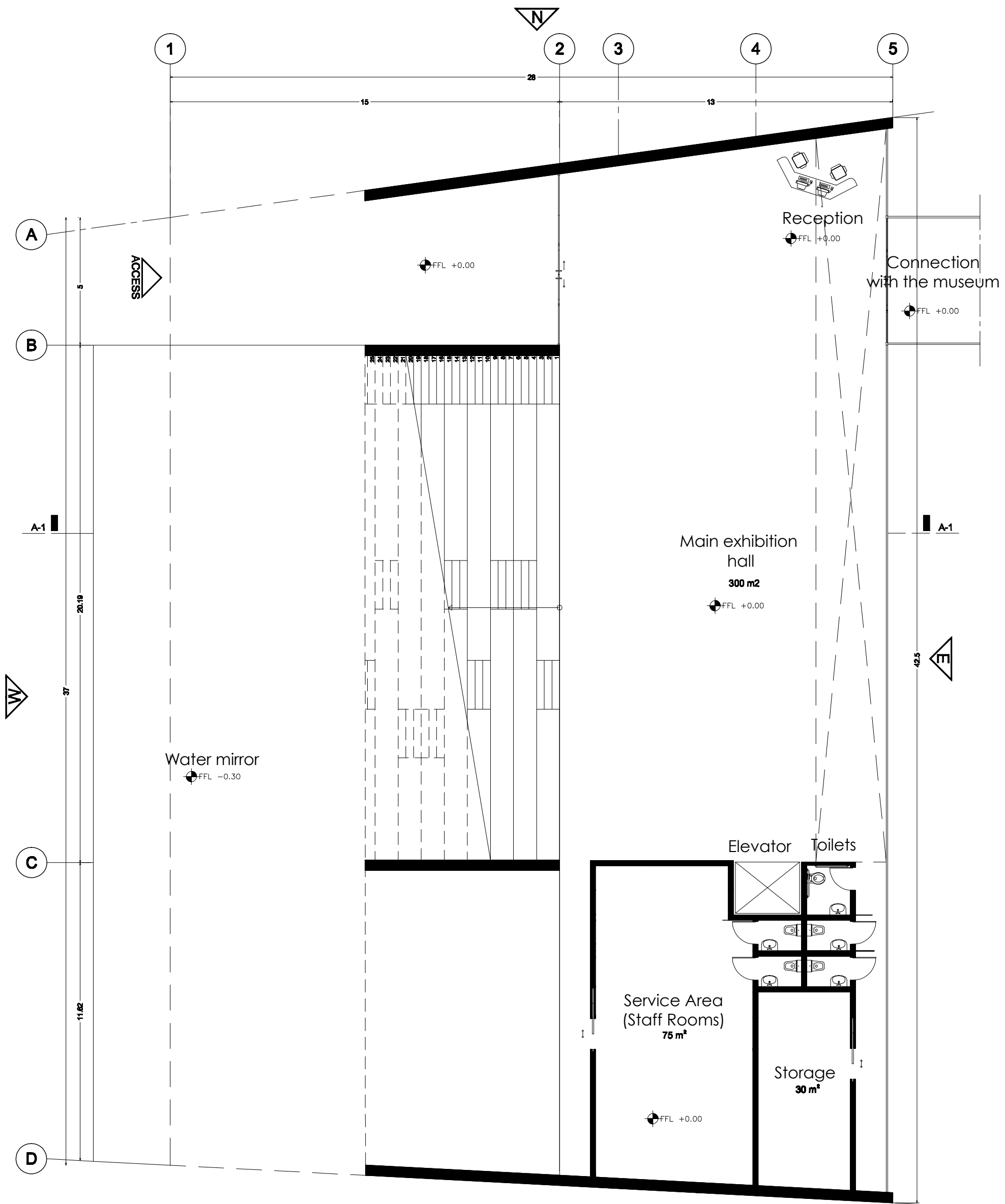
LEVEL 0 esc. 1:100
