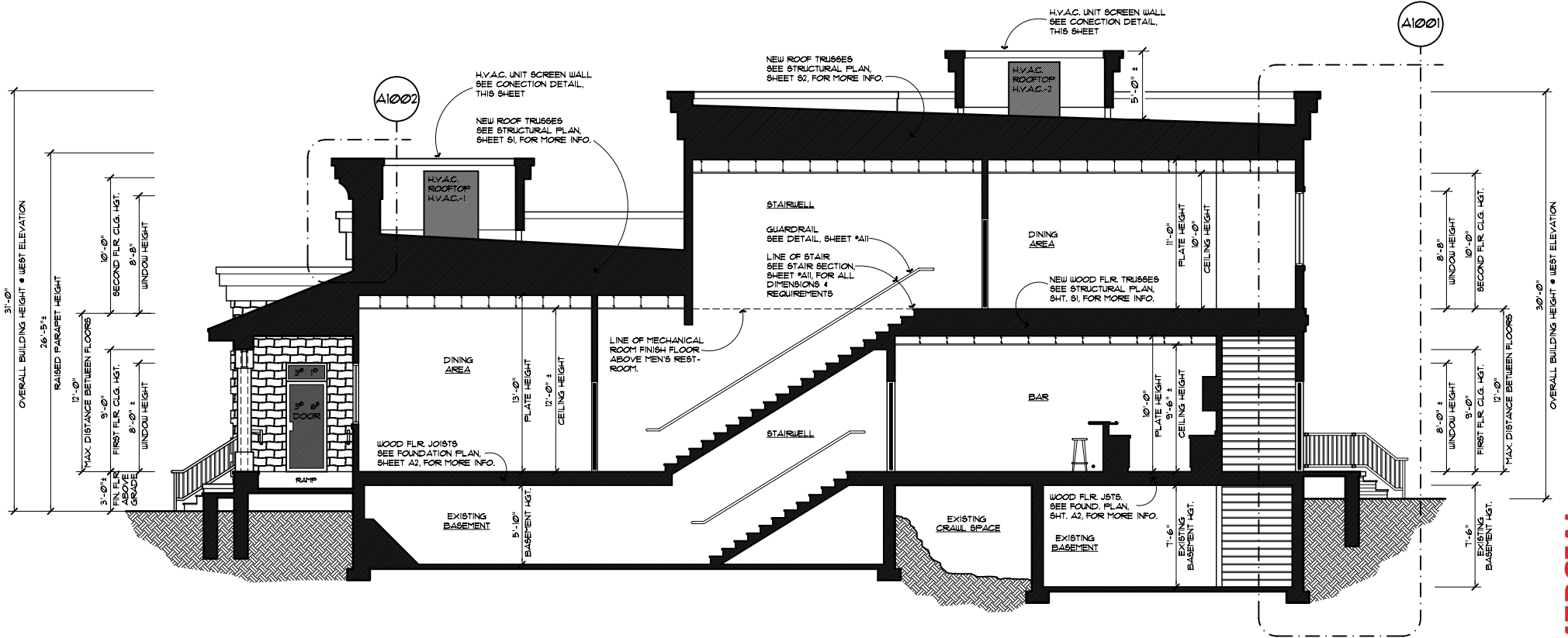
A801 A2, A3 A4, A5 BUILDING CROSS SECTION SCALE: 1/4" = 1'-0"
