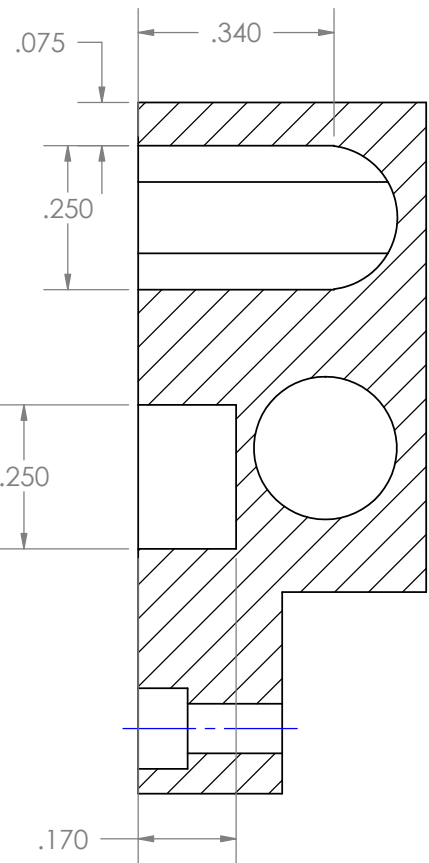
SECTION A-A SCALE 3 : 1
