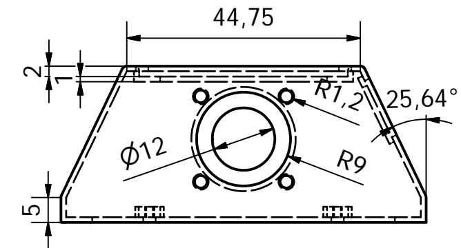
A-A (1 : 1)
