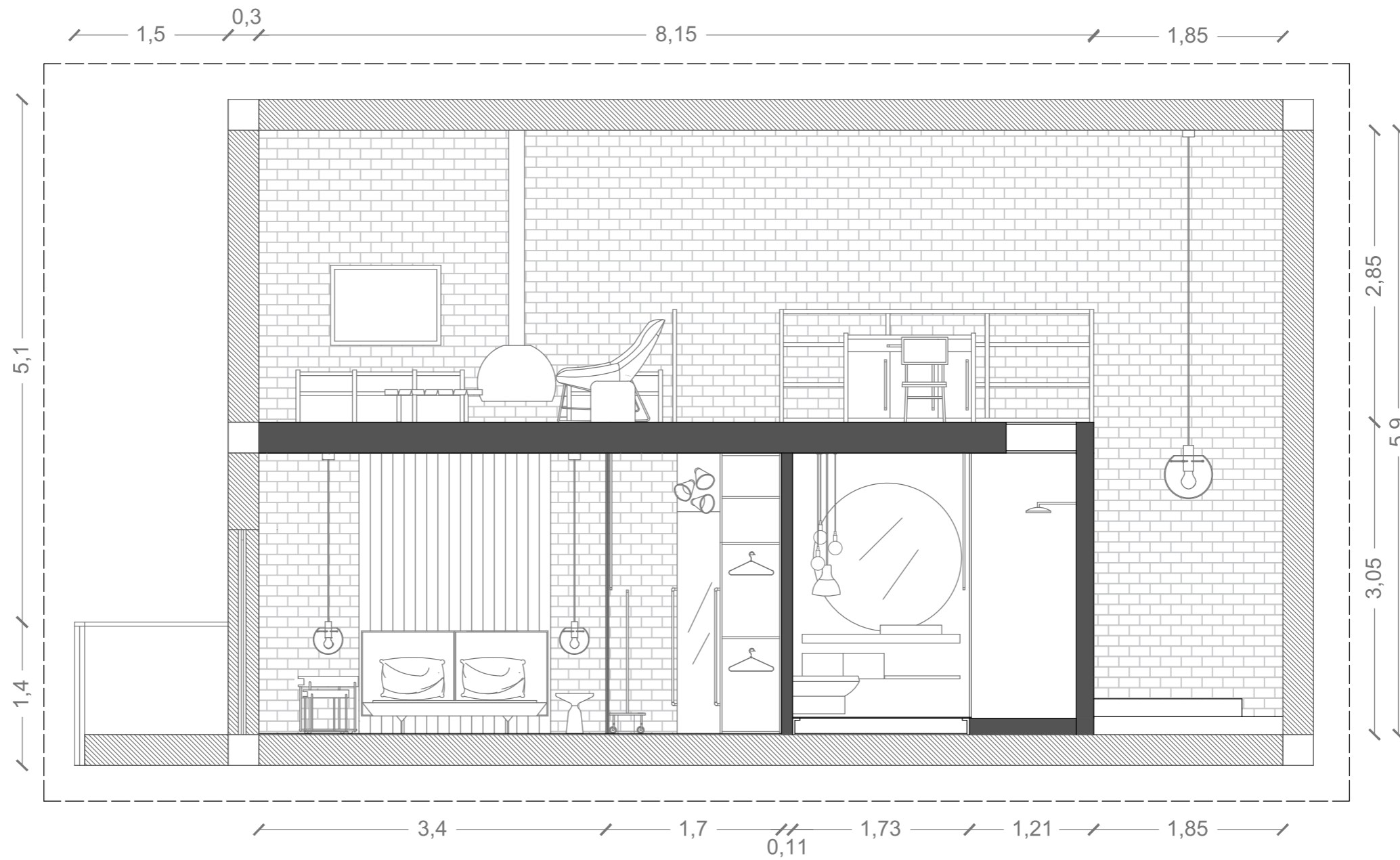
CORTE C-D
