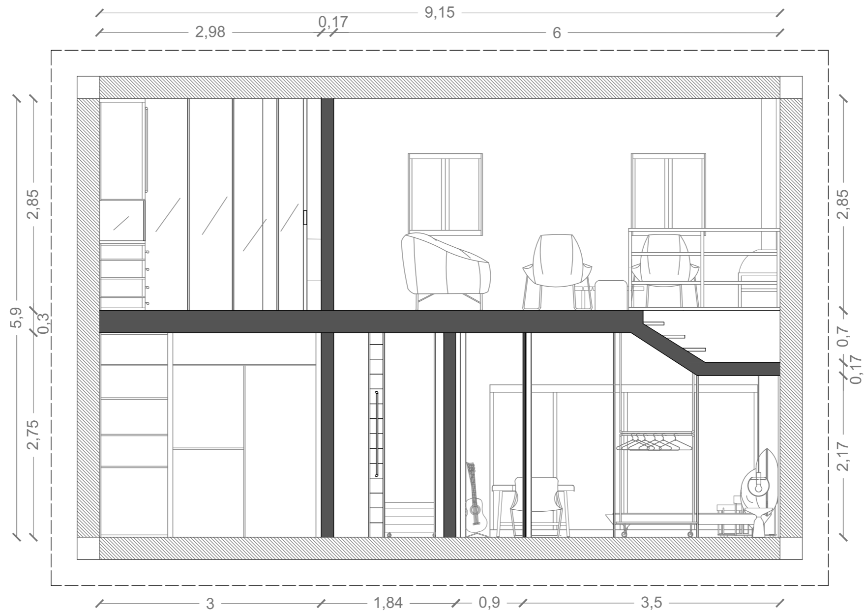
CORTE A-B
