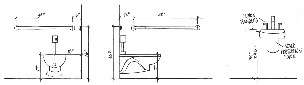
(D) A.D.A. LAVATORY ELEVATION
