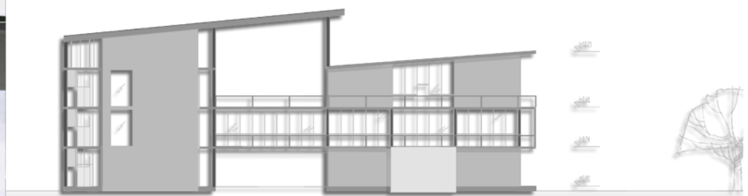
južna fasada R 1:200
