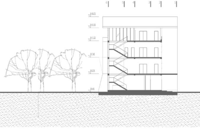
presek 1 - 1 R 1:200
