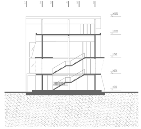
presek 2 - 2 R 1:200
