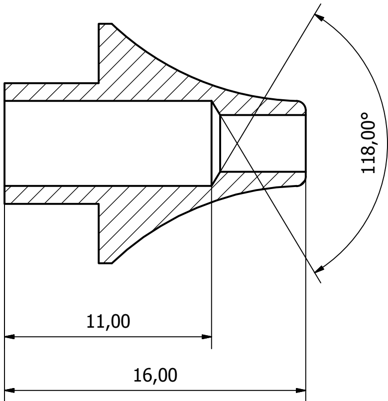
A-A ( 5 : 1 )
