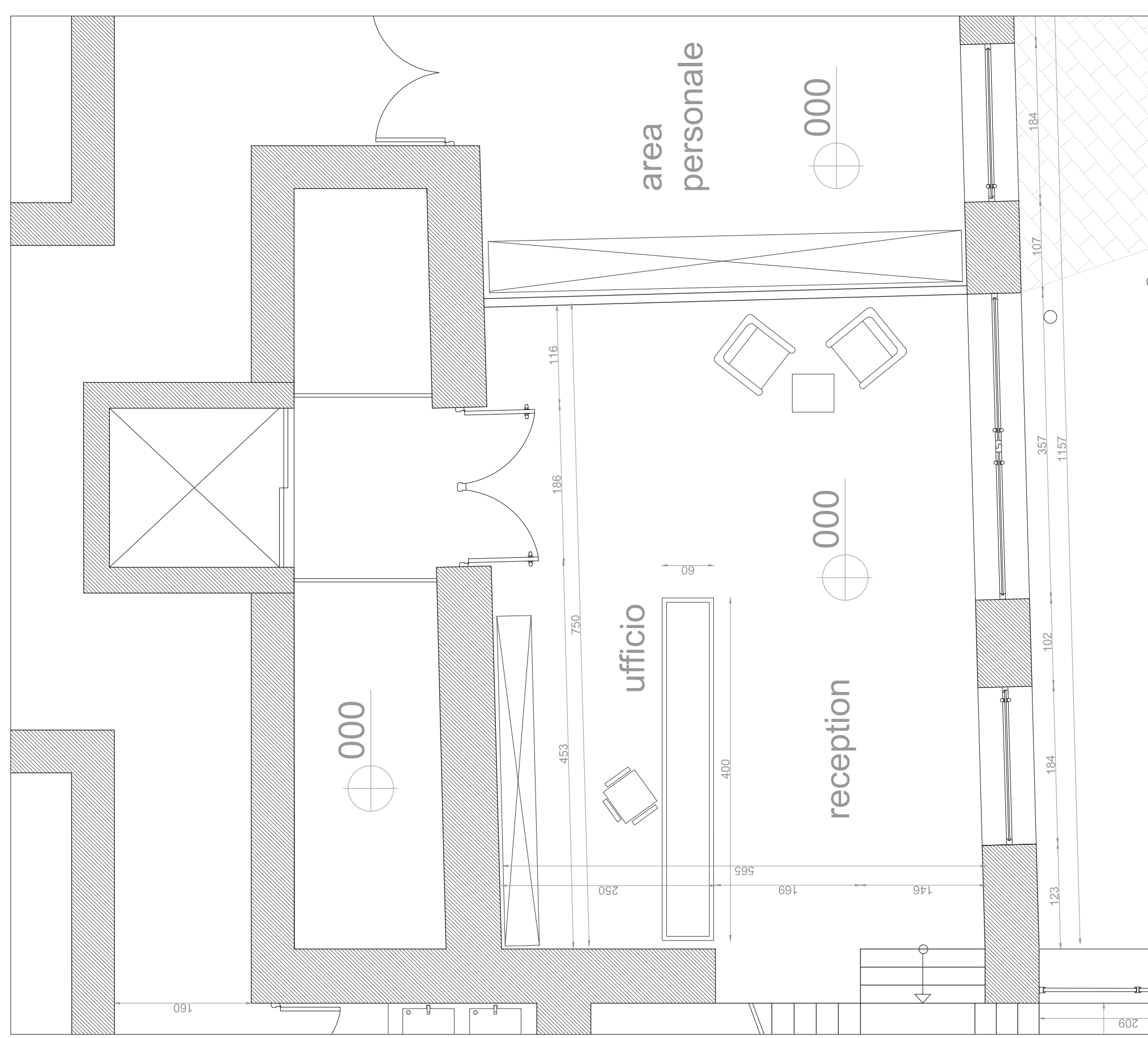
Particolare reception - scala 1.50
