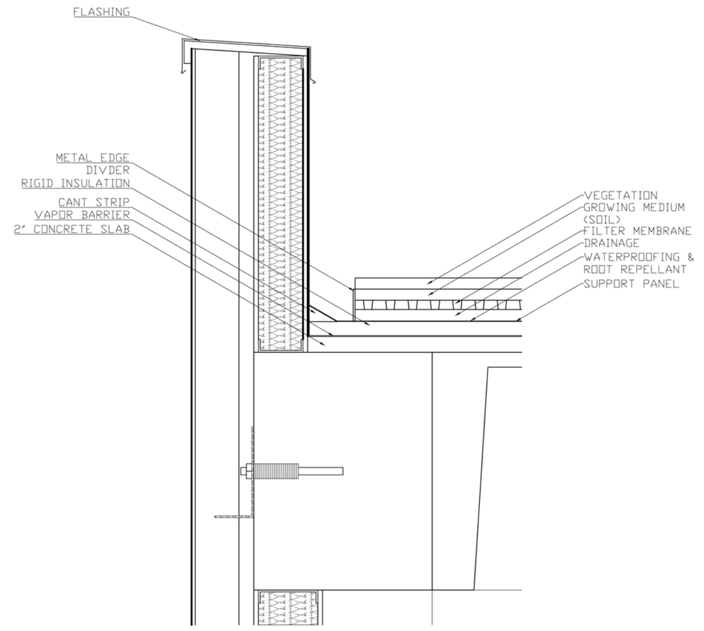
Detail One Scale: 1" = 1' - 0"
