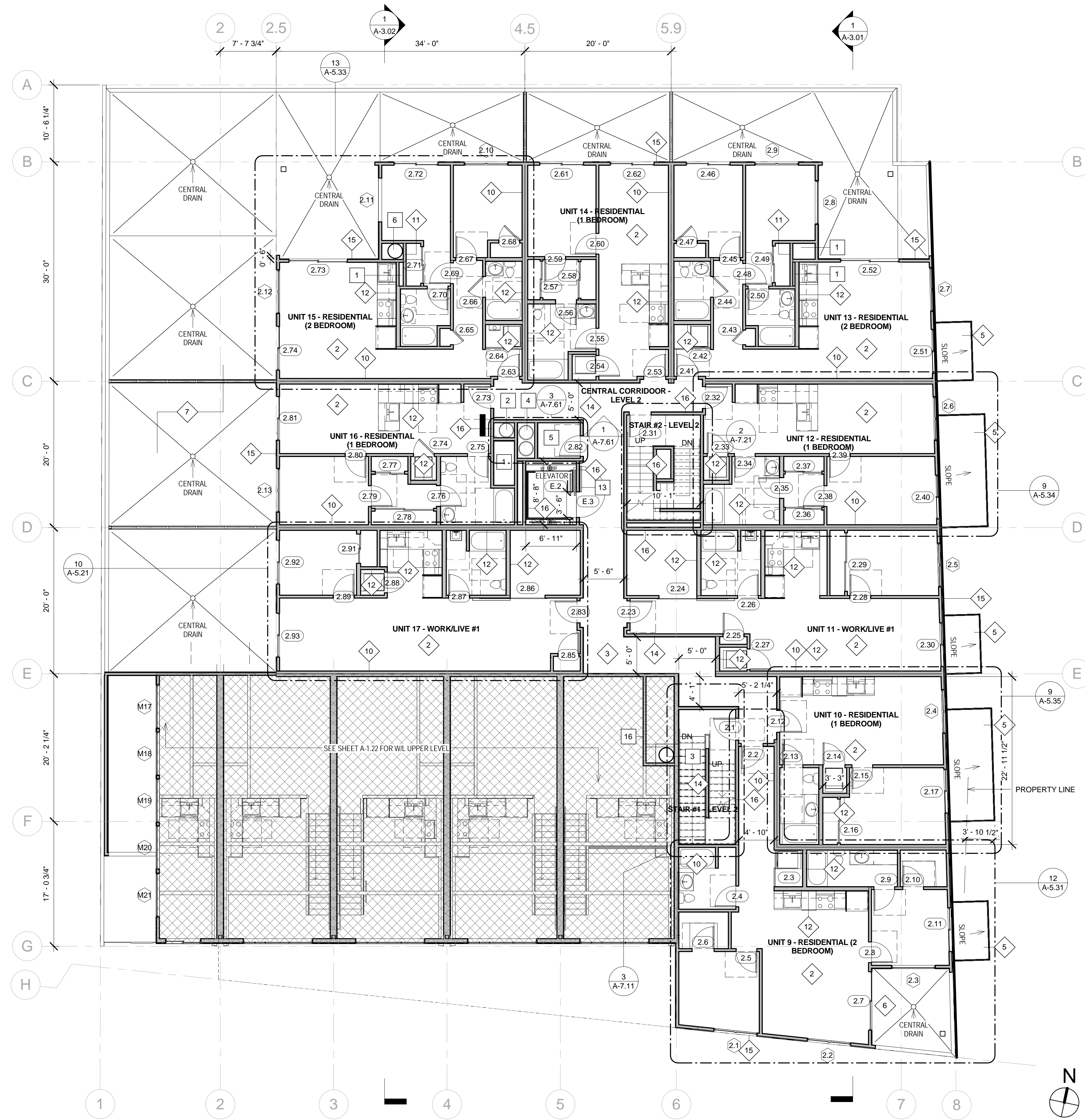
1 LEVEL 2 SCALE: 1/8" = 1'-0"
