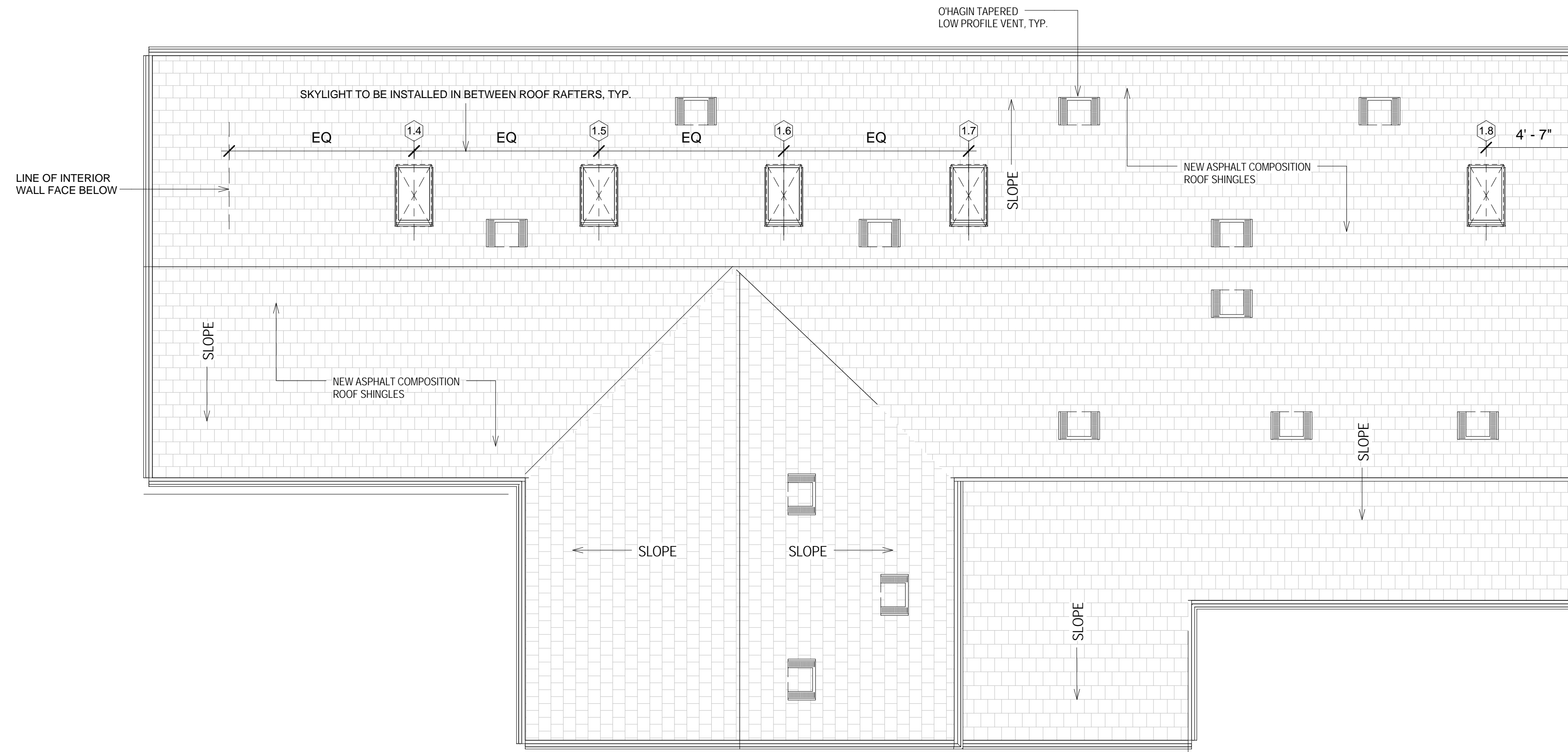
2 (3320) ROOF SCALE: 1/4" = 1'-0"
