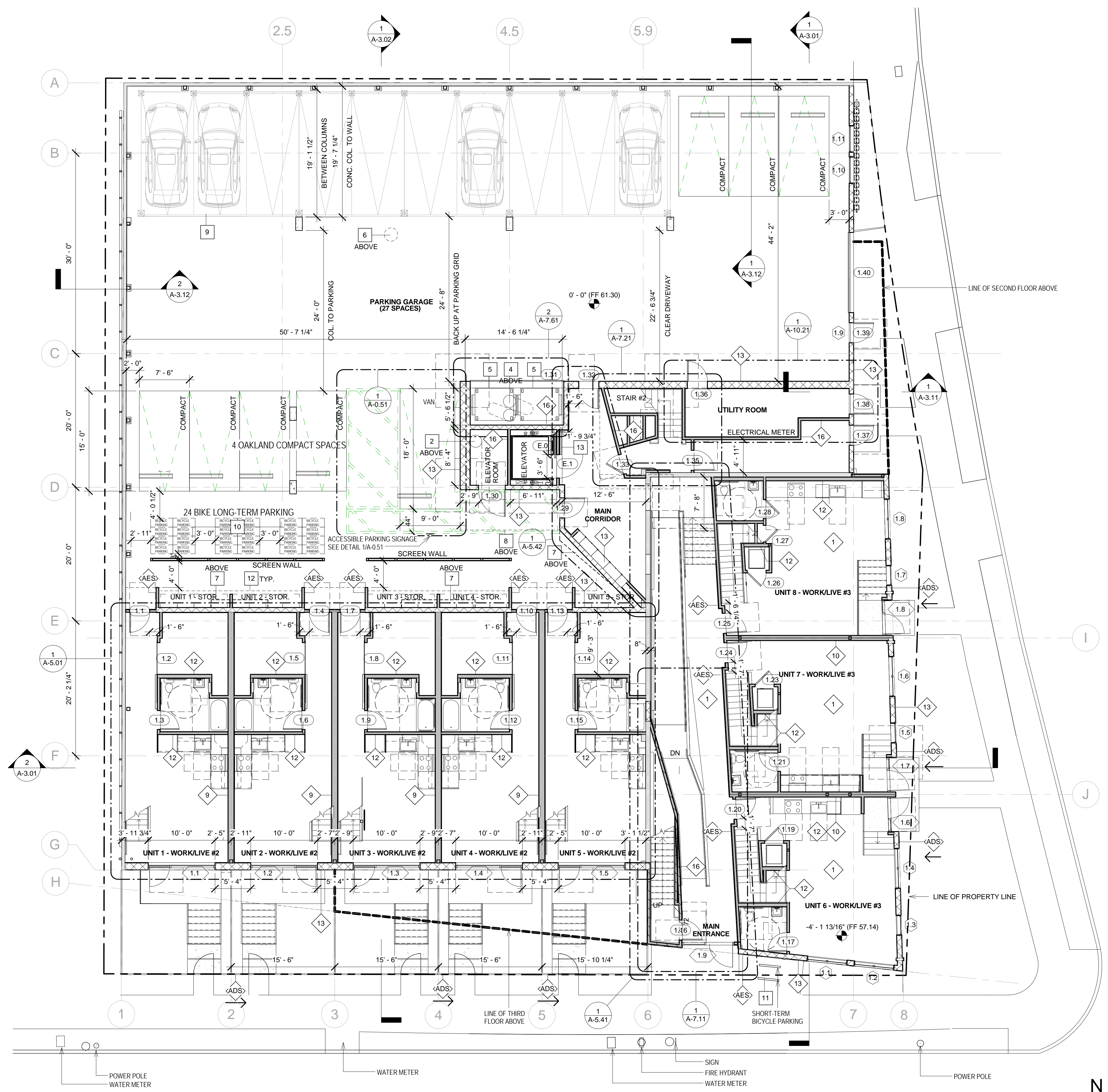
1 LEVEL 1 SCALE: 1/8" = 1'-0"
