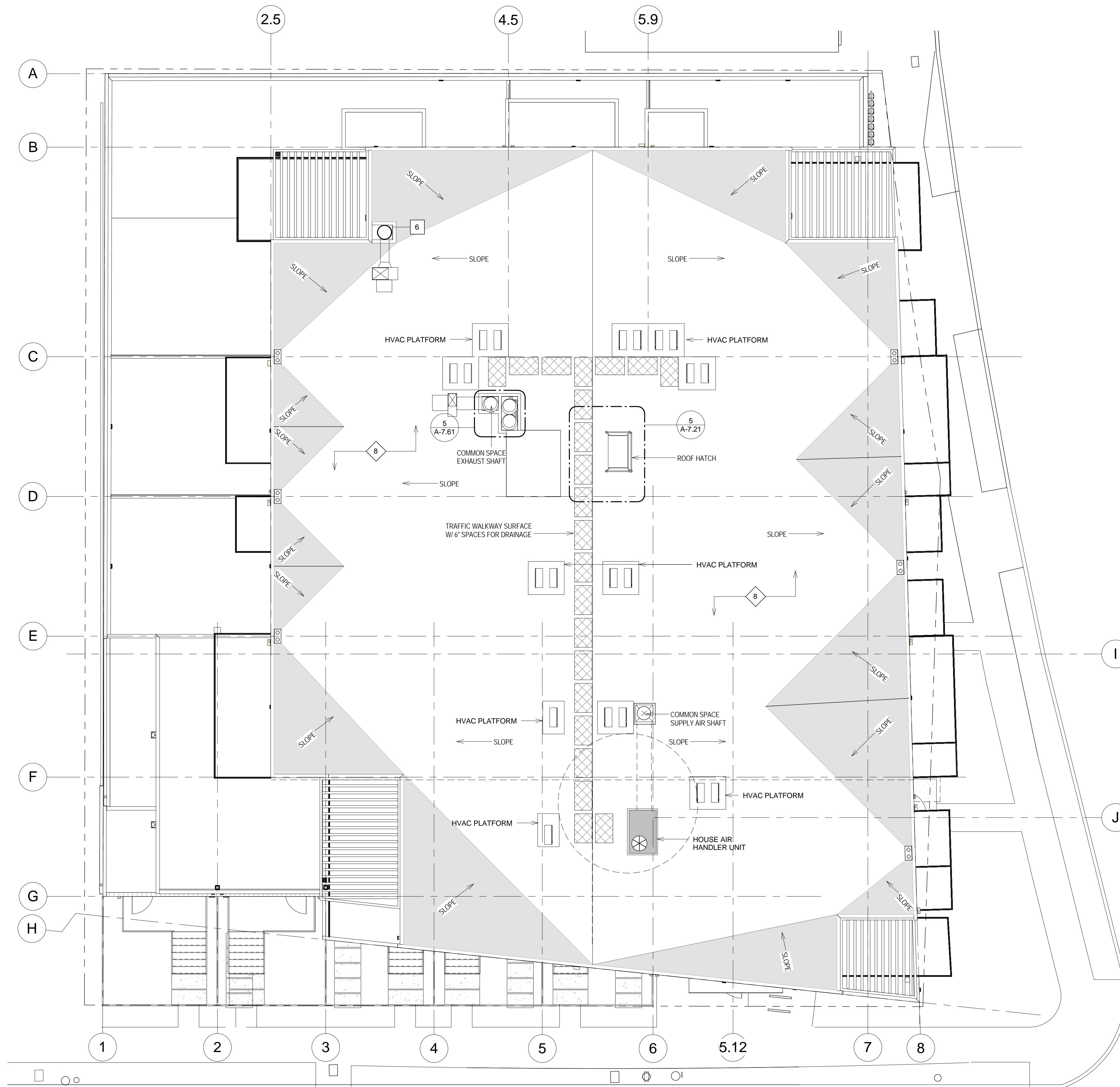
1 ROOF SCALE: 1/8" = 1'-0"
