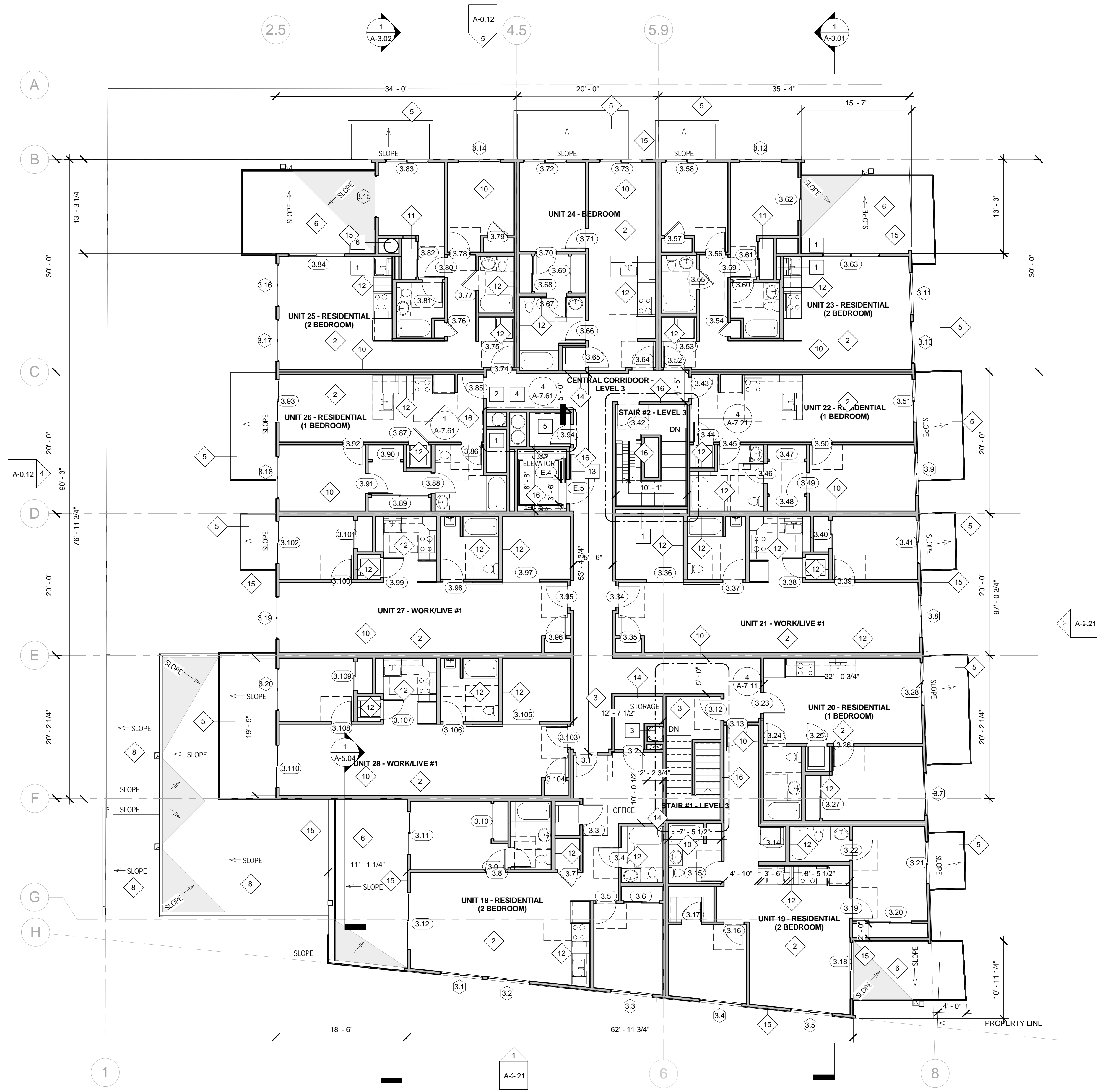
1 LEVEL 3 SCALE: 1/8" = 1'-0"
