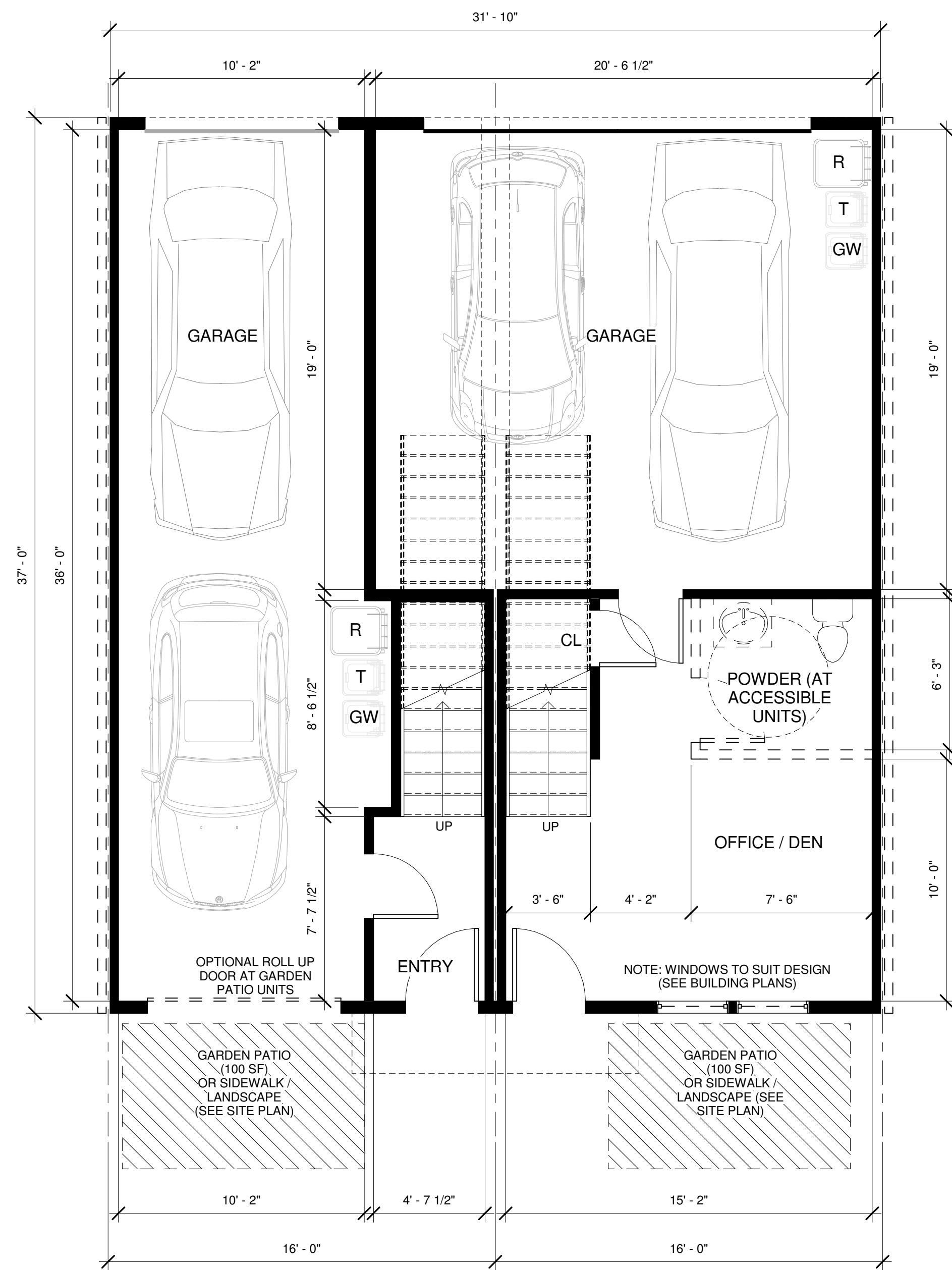
1 UNIT A1/B1 LEVEL 1 SCALE: 1/4" = 1'-0"
