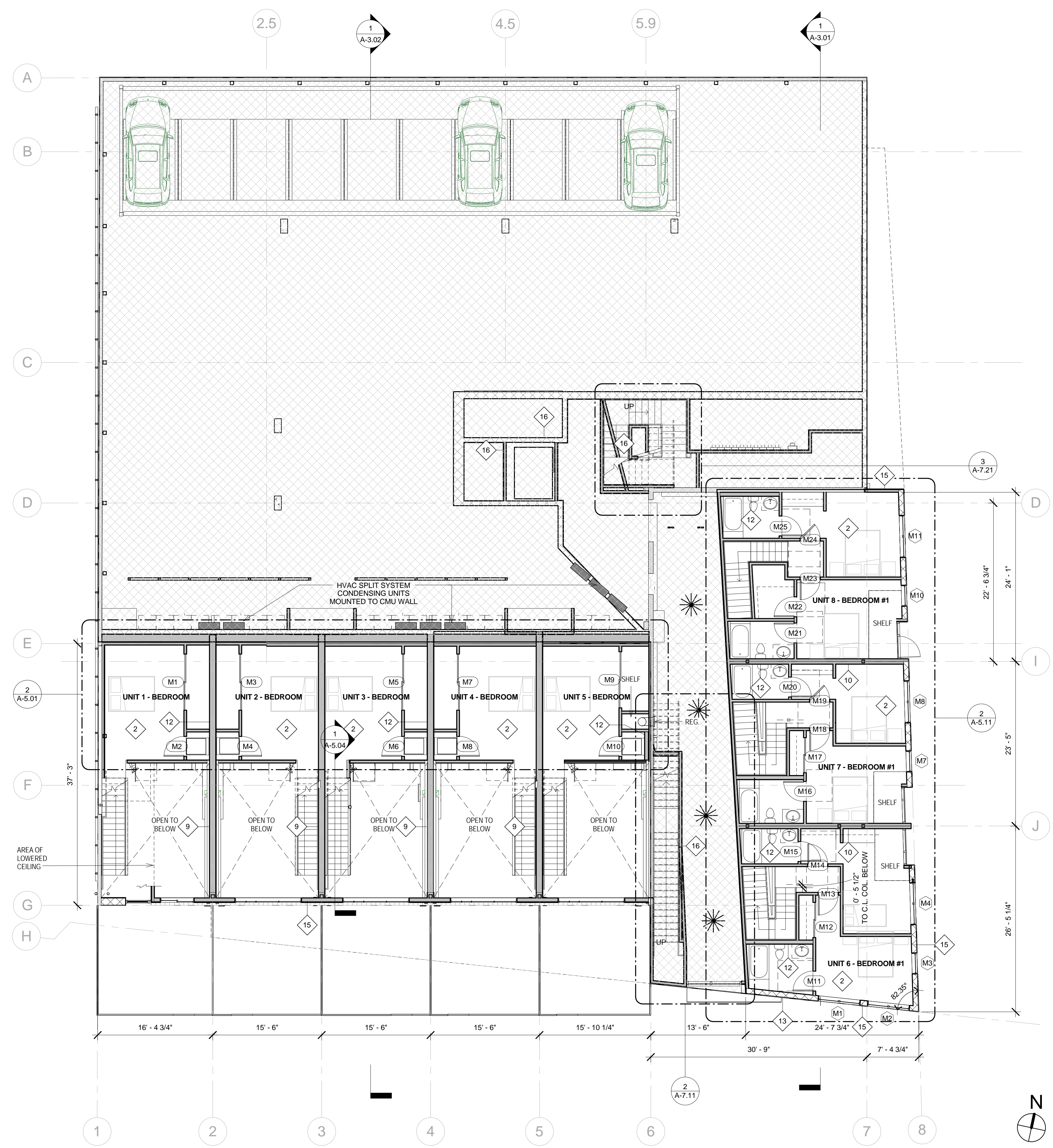
1 LEVEL 1.5 SCALE: 1/8" = 1'-0"
