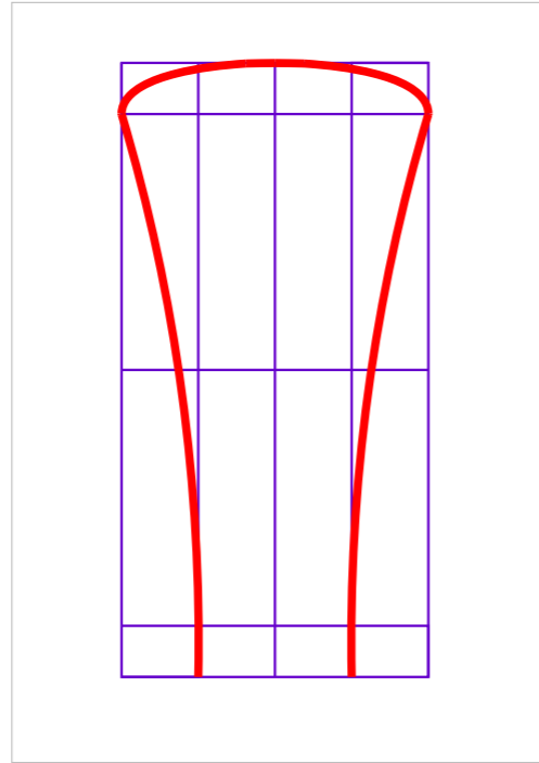
Parábola Conoídica
