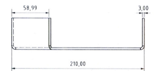
Part 2 - MTS330_Base-p1 ( 1 : 2 )
