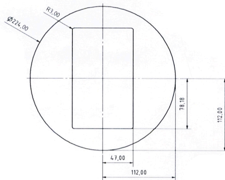
Part 1 ( 1 : 2 )
