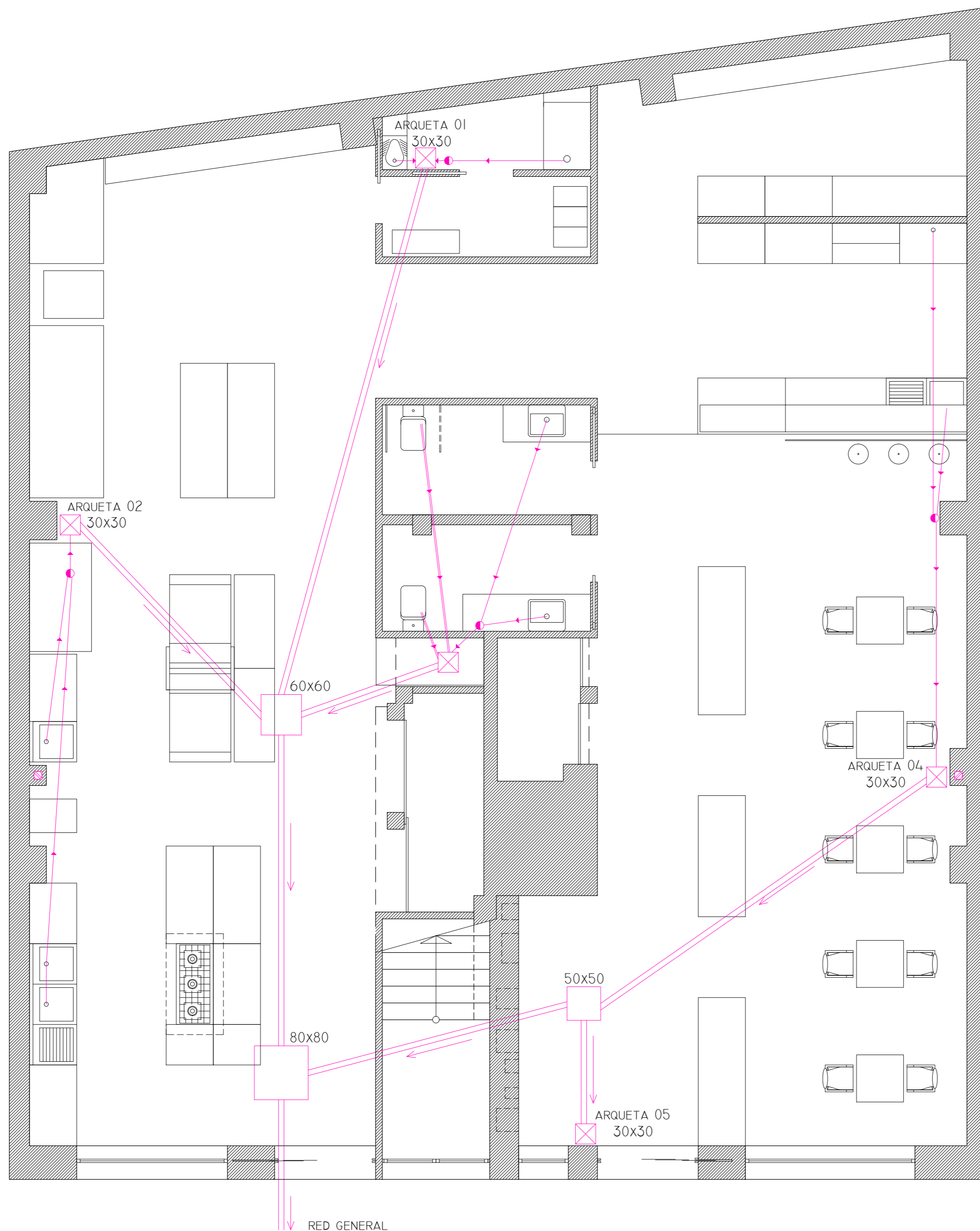
PLANTA ESQUEMA INSTALACIÓN SANEAMIENTO.
