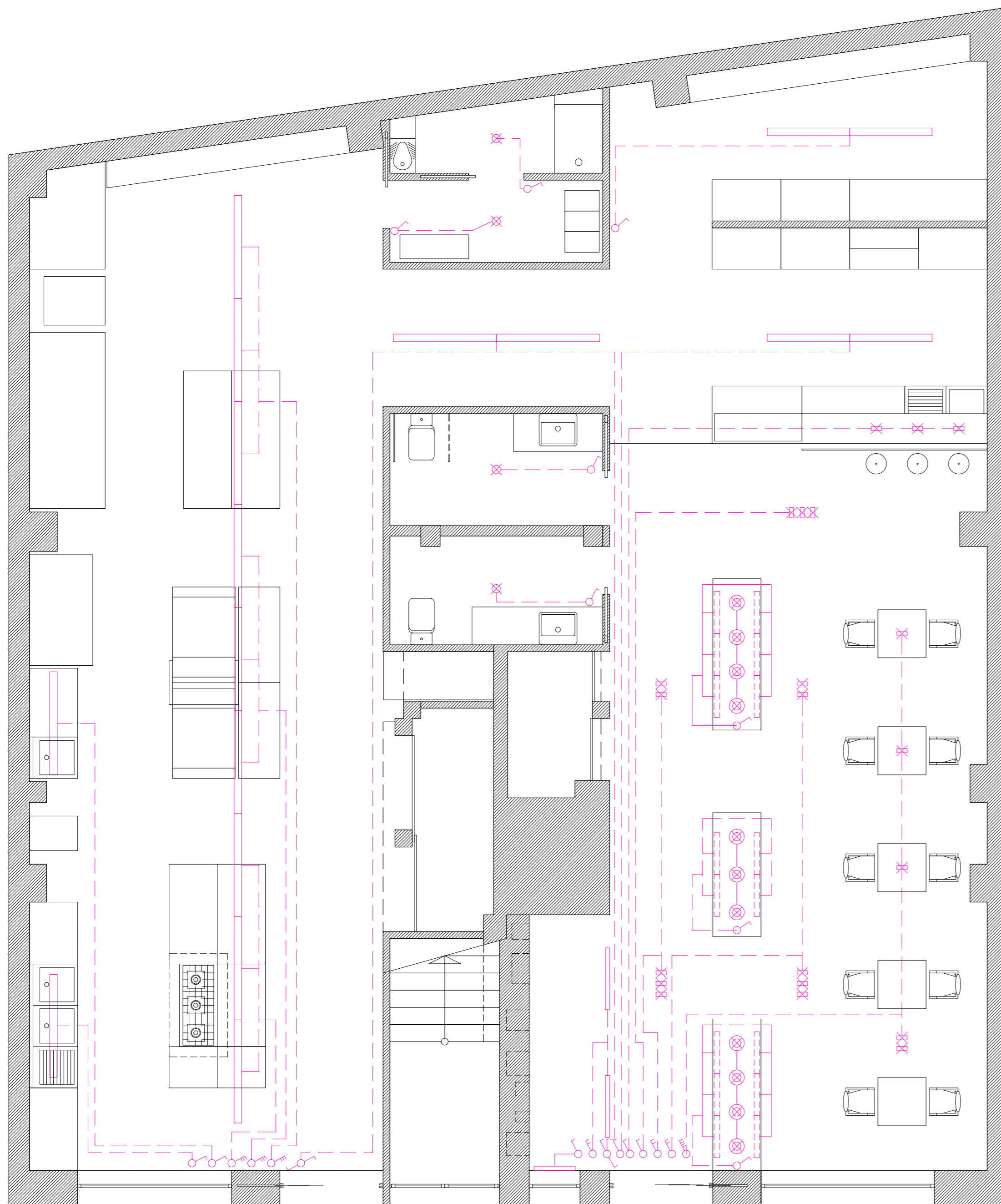
PLANTA ESQUEMA INSTALACIÓN ILUMINACIÓN.
