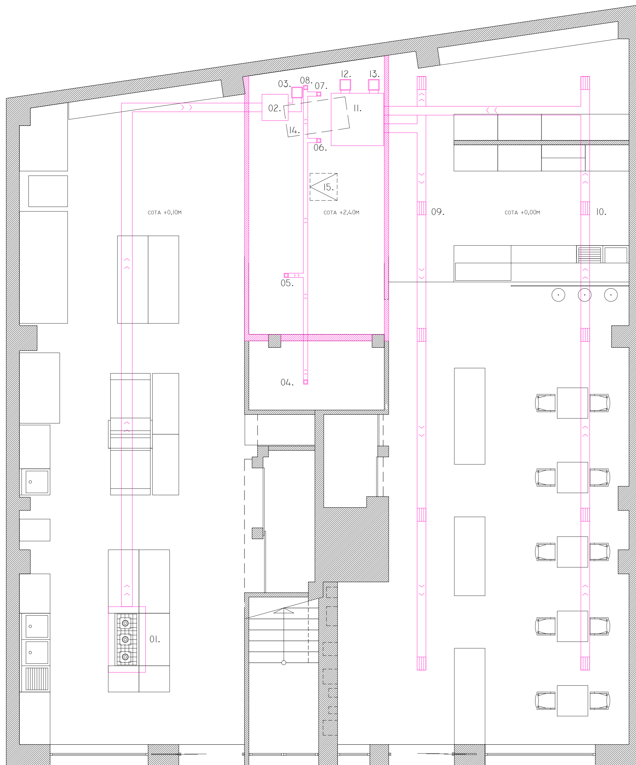
PLANTA ESQUEMA INSTALACIÓN CLIMATIZACIÓN, EXTRACCIÓN Y VENTILACIÓN.
