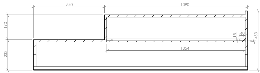
SECCIÓN S-S ESCALA 1 : 15
