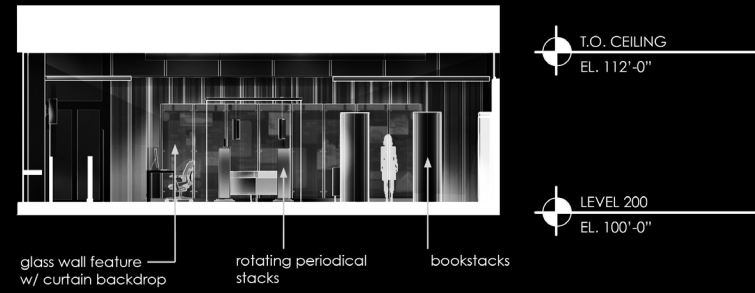
A latitudinal section 1/8" = 1'-0"
