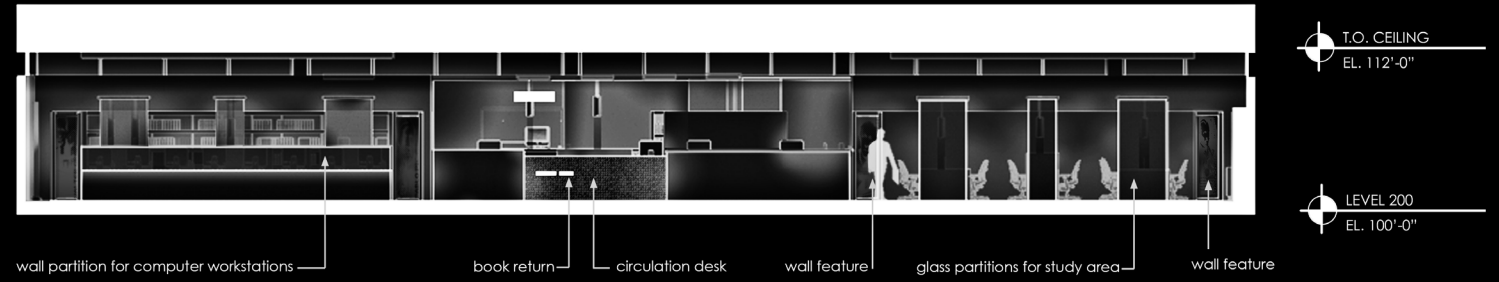
B longitudinal section 1/8" = 1'-0"
