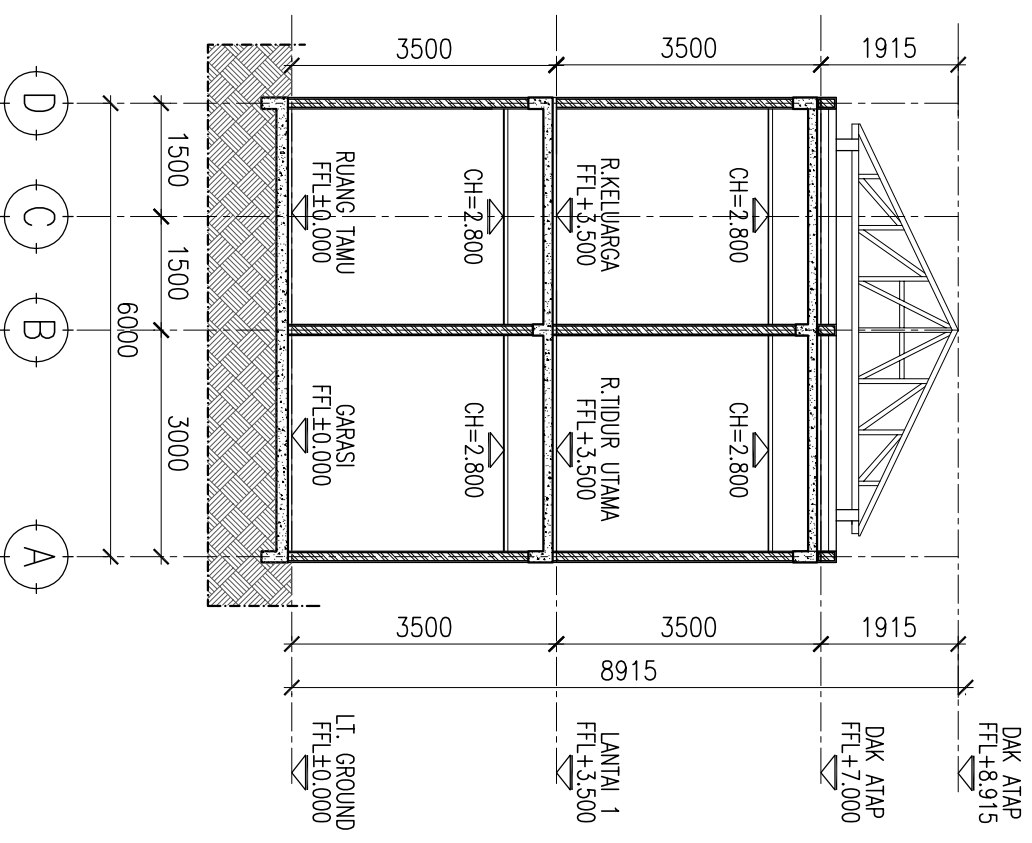
2 POTONGAN B A1-002 SCALE 1 : 100
