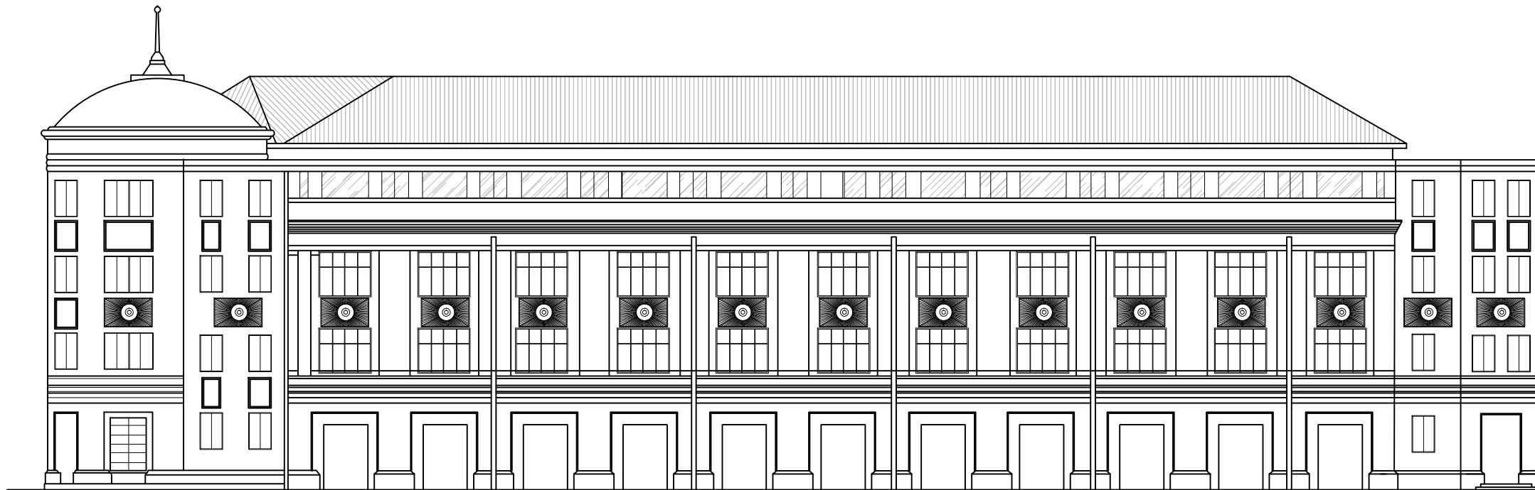
ELE 1.1 1:250
