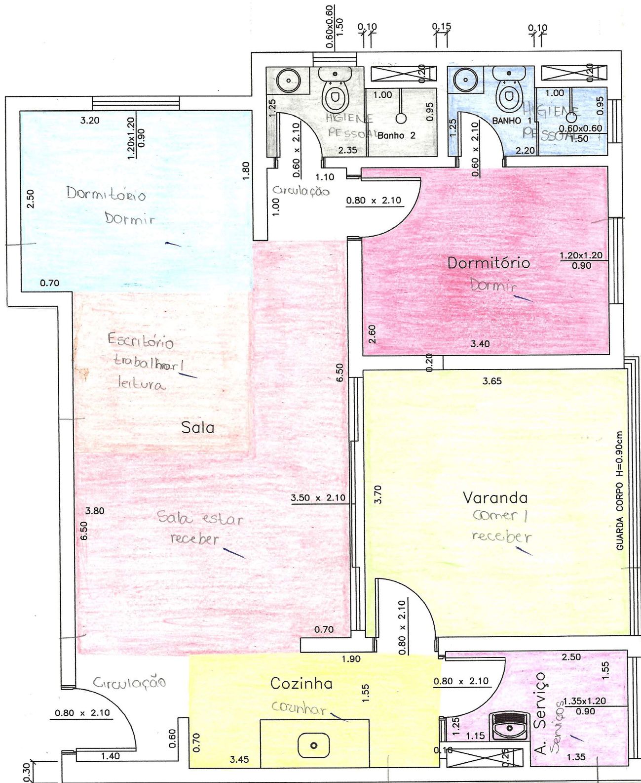
PLANTA Esc 1/50
