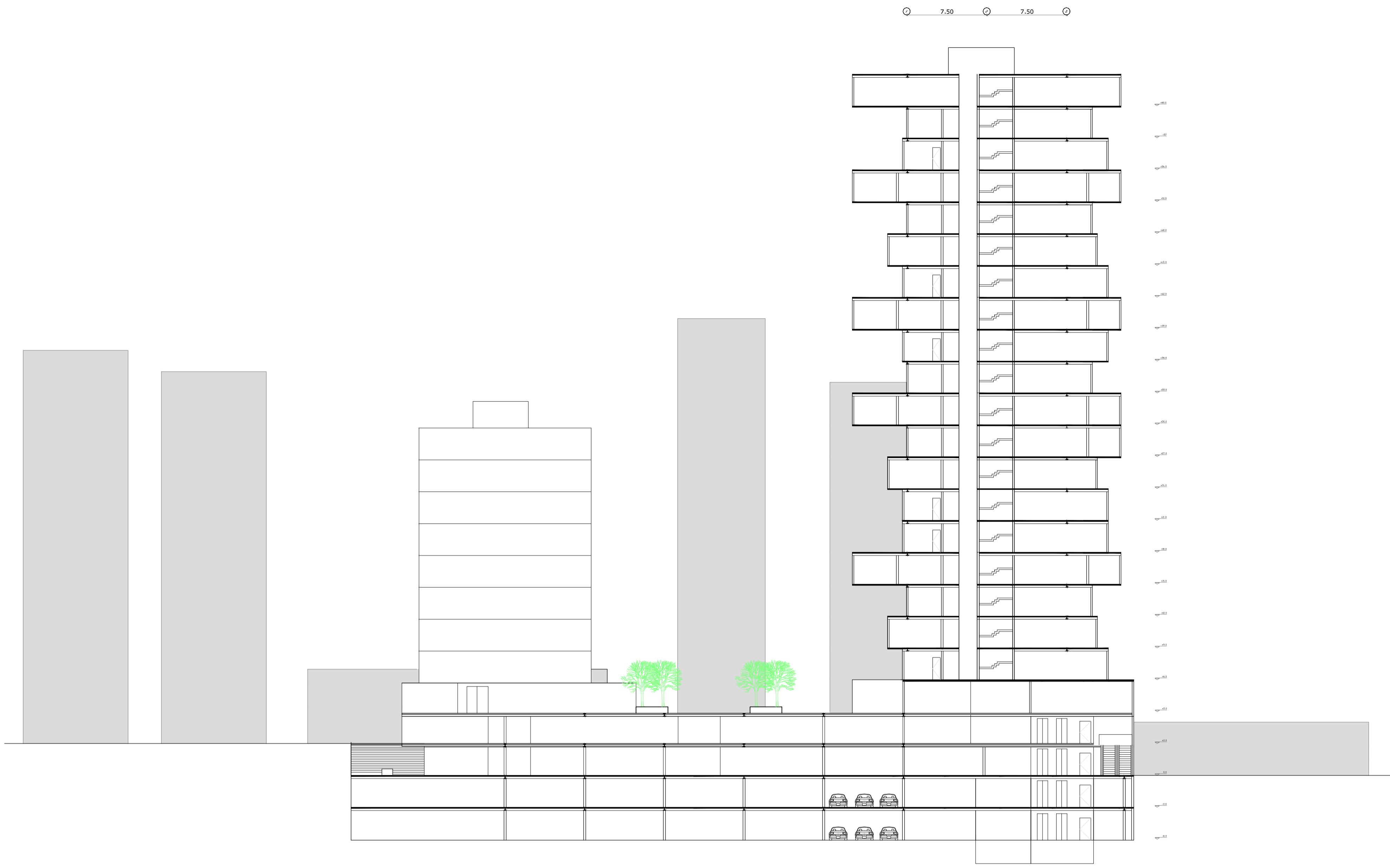
CORTE C.C
