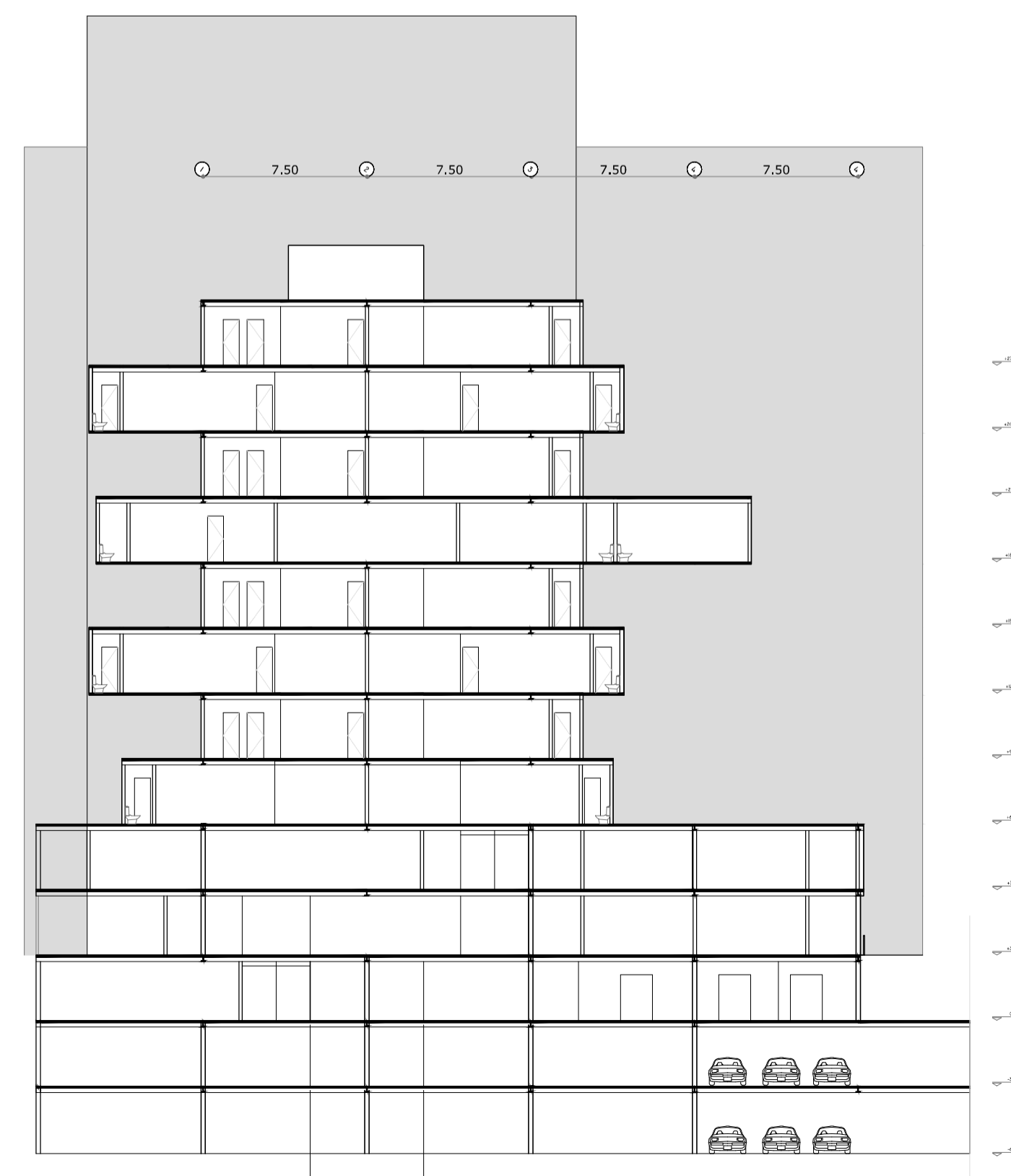
CORTE C.C
