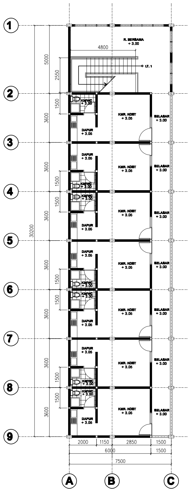
DENAH LANTAI. 1
