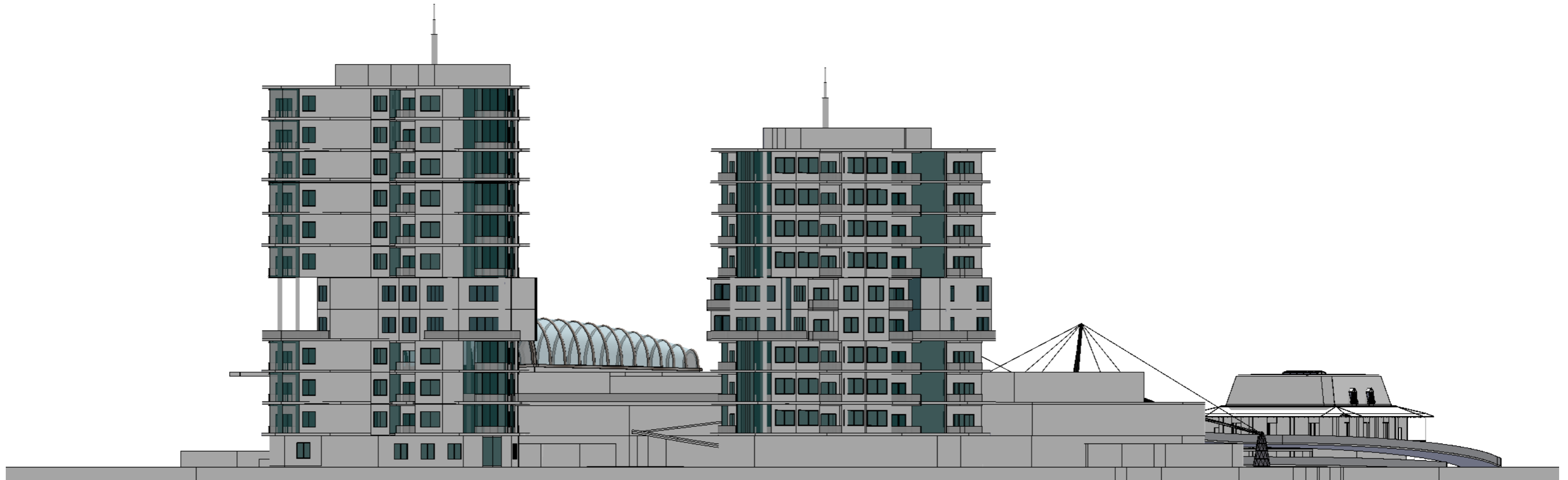
TAMPAK BELAKANG SKALA 1:500
