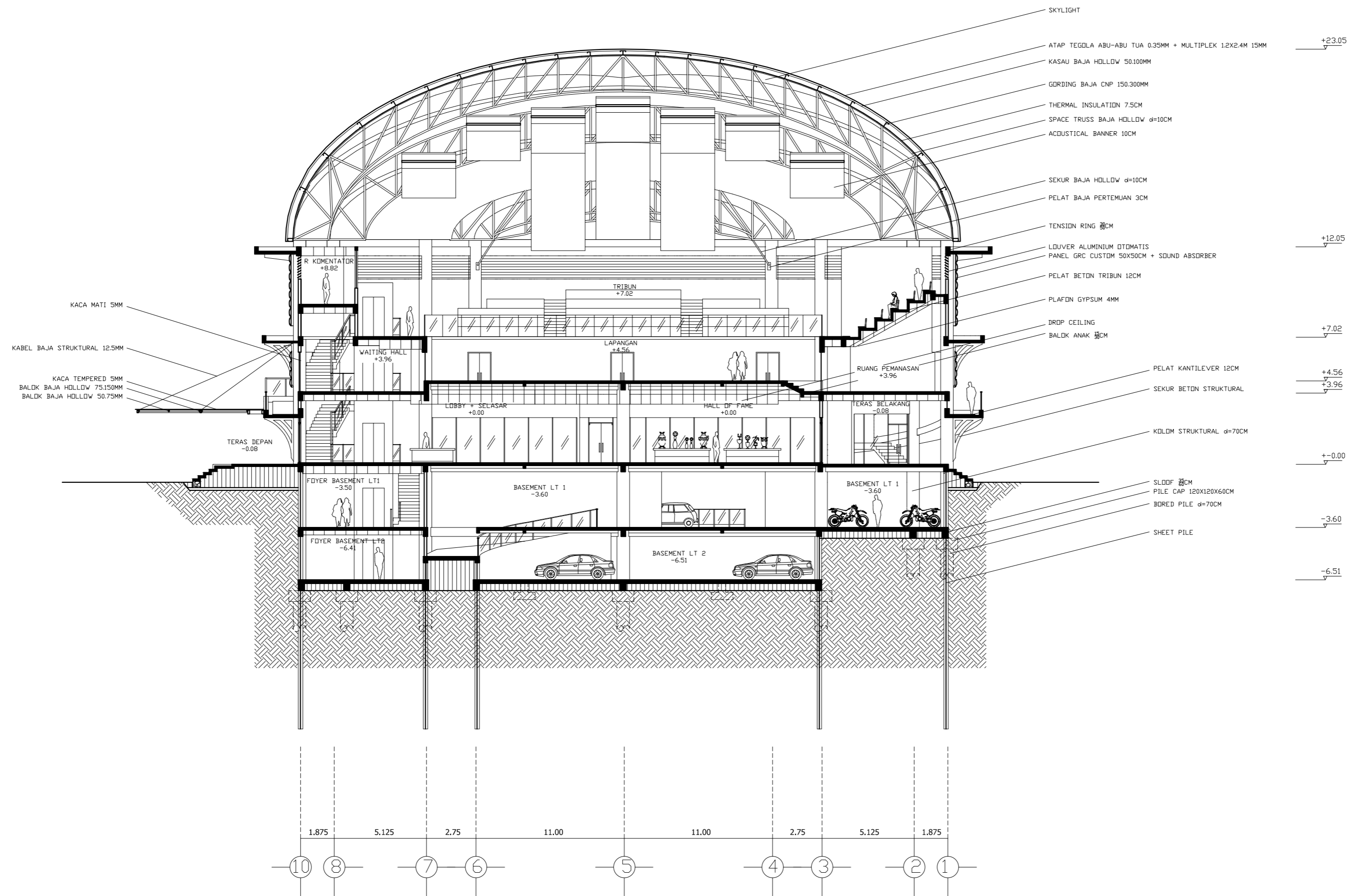
POTONGAN II-II' SKALA 1 : 200
