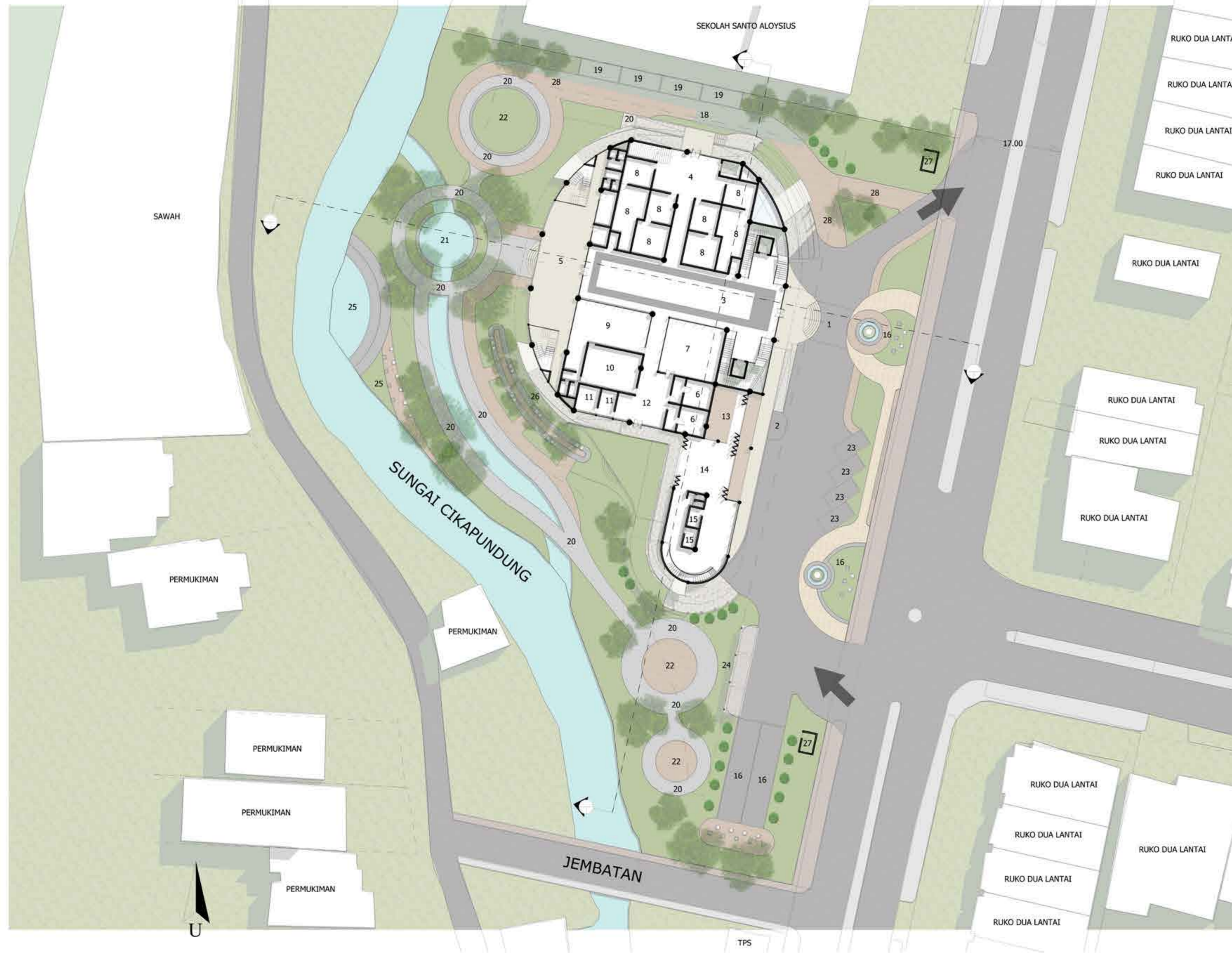
SITE PLAN SKALA 1 : 400
