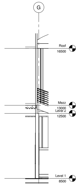
1 Wall Section 1 1 : 50
