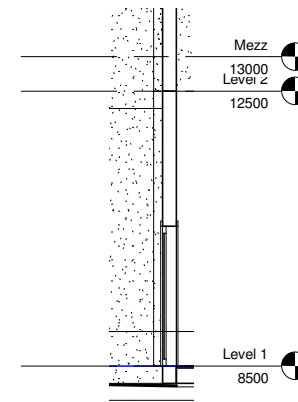
2 Wall Section 2 1 : 50
