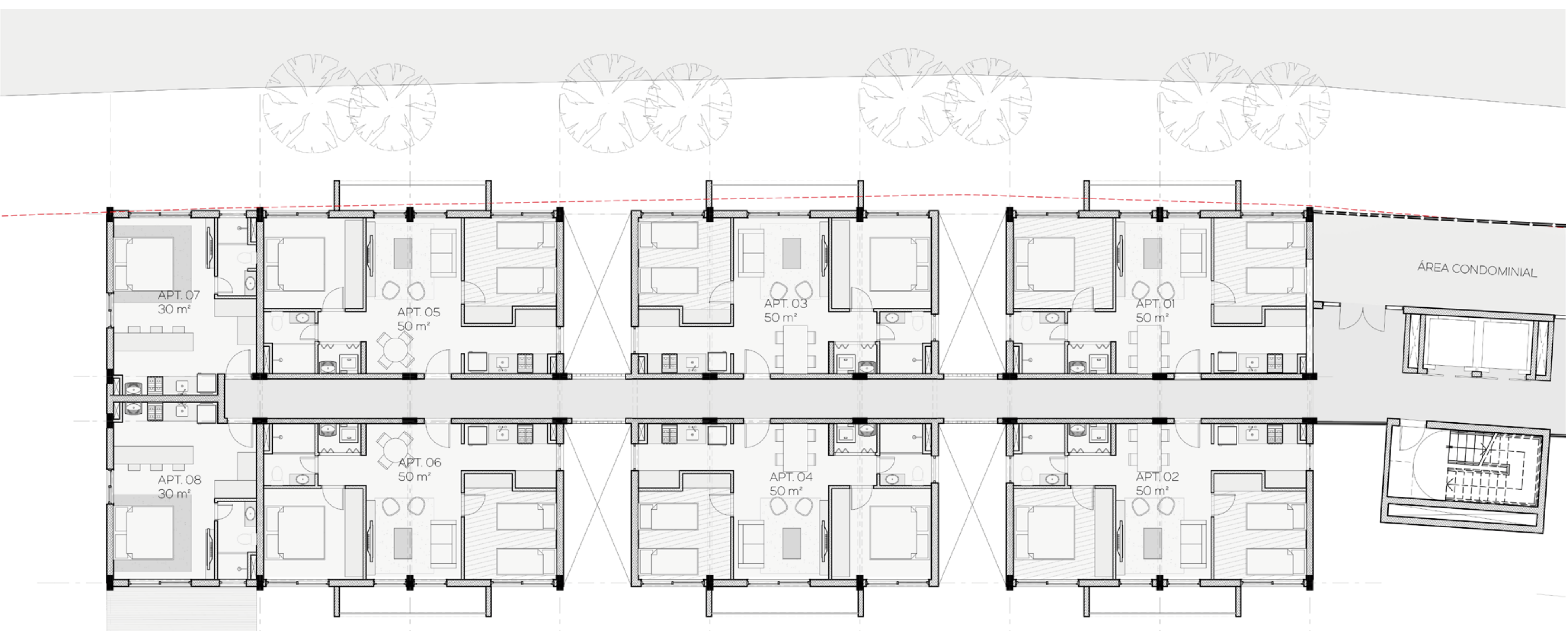
PLANTA BAIXA PAV. TIPO RESIDENCIAL esc: 1/100
