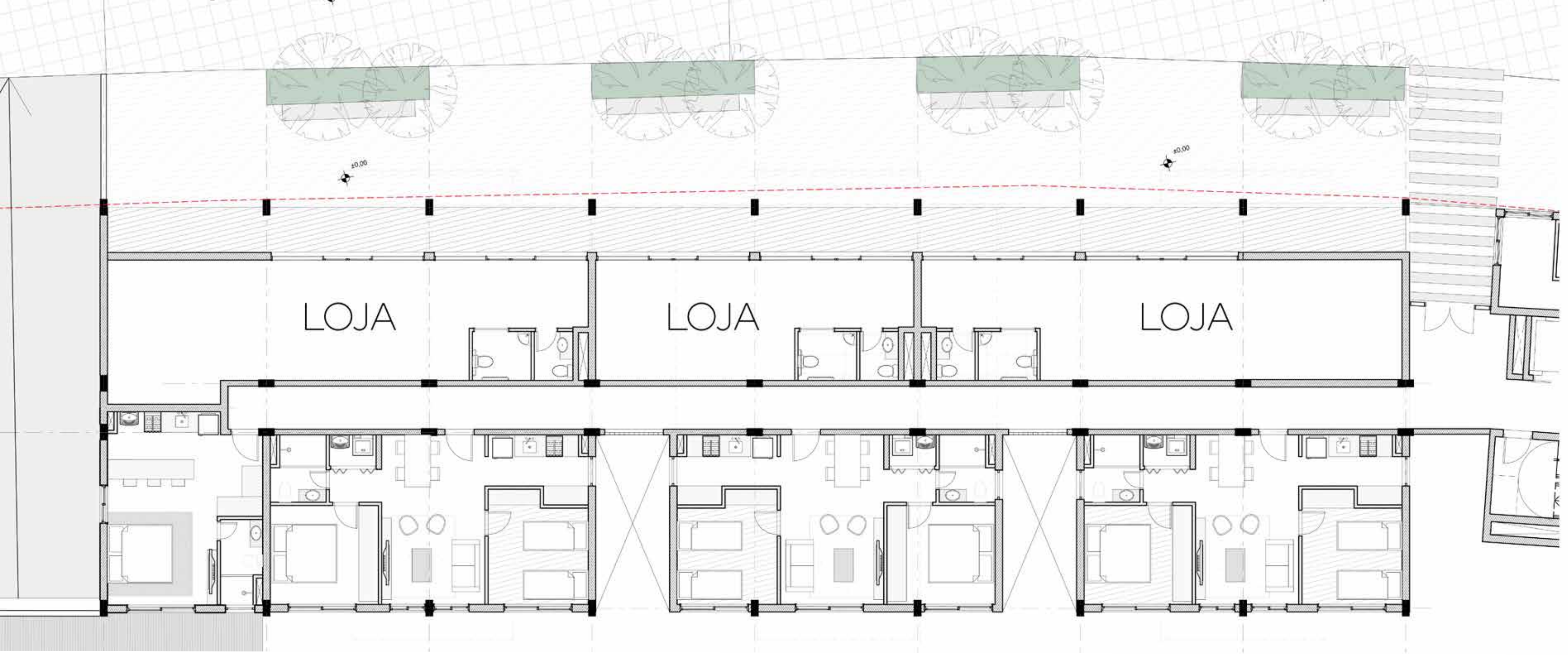
PLANTA BAIXA PAV. TIPO RESIDENCIAL esc: 1/100
