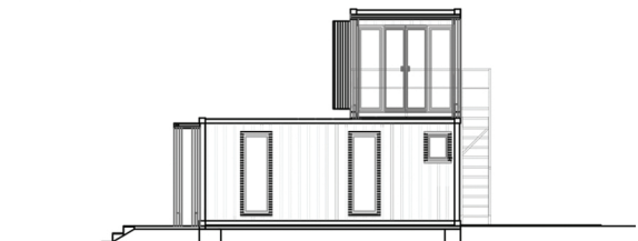
06 RIGHT ELEVATION
