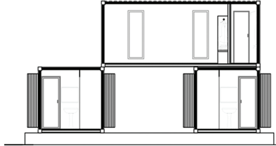
08 SECTION BB
