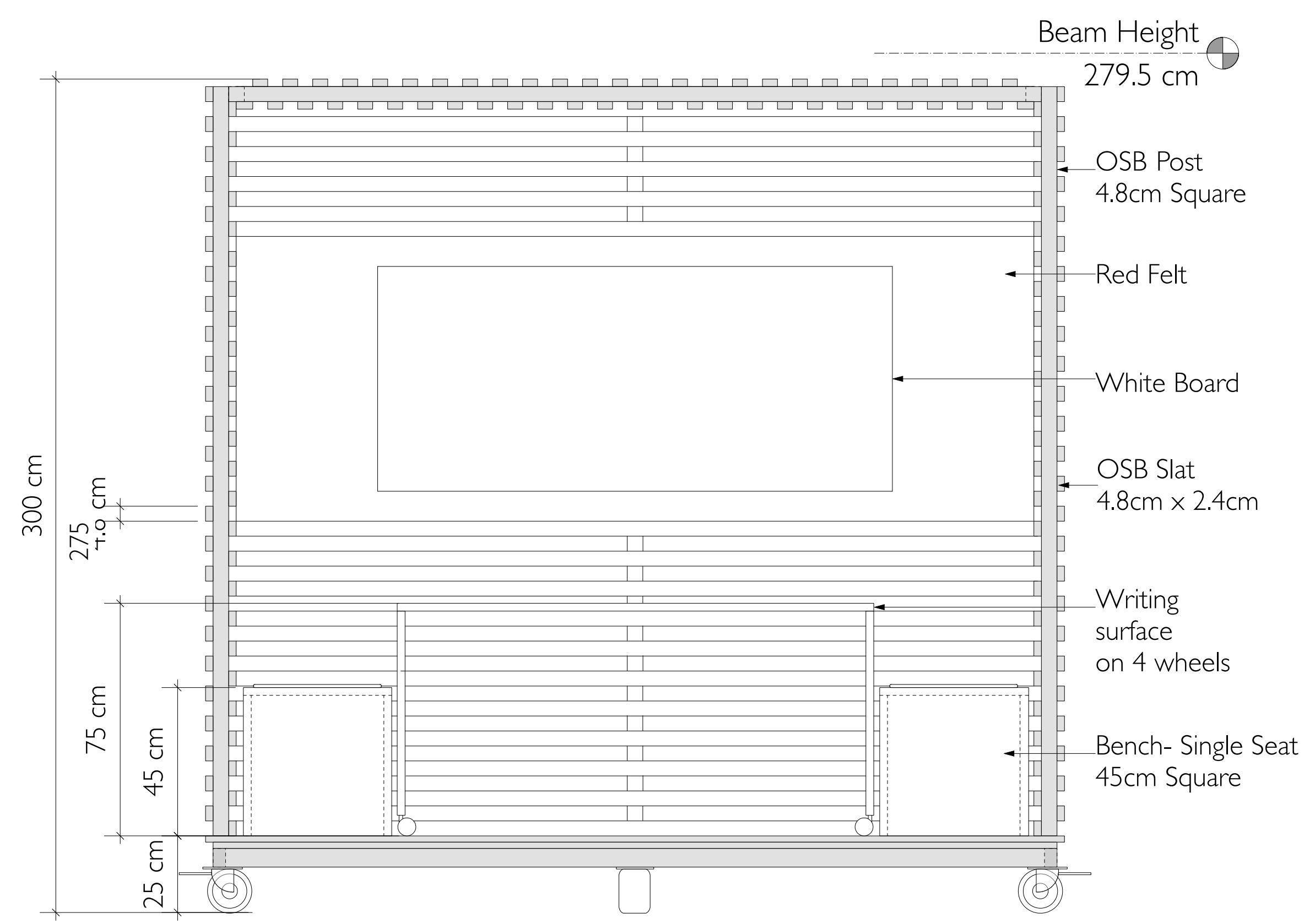
THINKTANK SECTION 1:15
