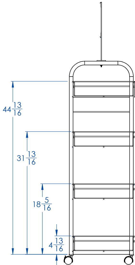
SECTION A-A
