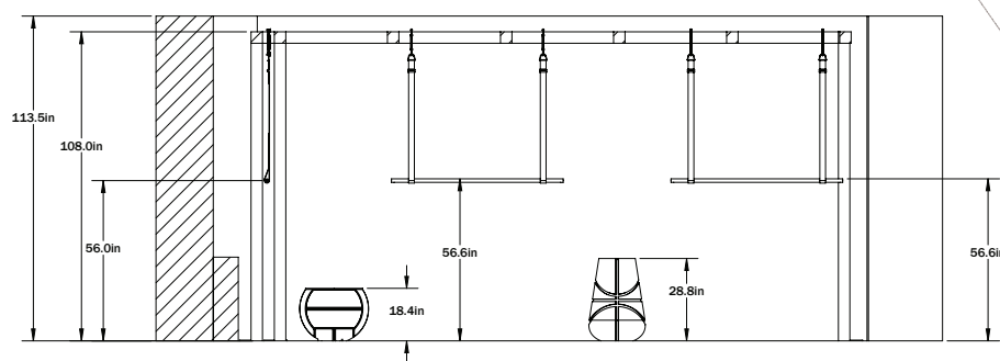
SECTION A-A SCALE 1 : 32
